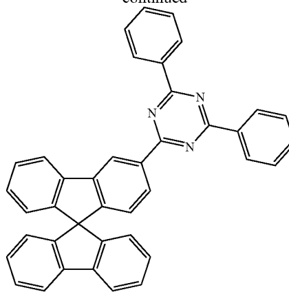
SF3-TRZ
