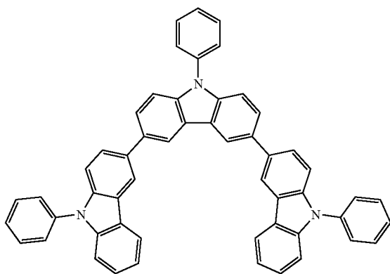
Tris-PCz
