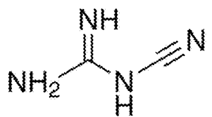
Dicyandiamide (DCDA)
