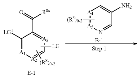
Scheme-13:
