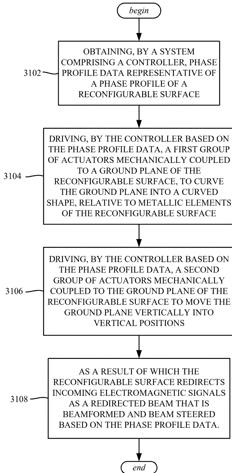
FIG. 31
