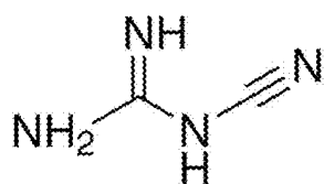
Dicyandiamide (DCDA)
