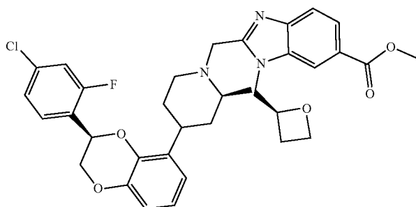
Methyl 2-(((2S)-4-((R)-3-(4-chloro-2-fluorophenyl)-2,3-dihydrobenzo[b][1,4]dioxan-5-yl)-2-methylpiperidin-1-yl)methyl)-1-(((S)-oxetan-2-yl)methyl)-1H-benzo[d]imidazole-6-carboxylate
