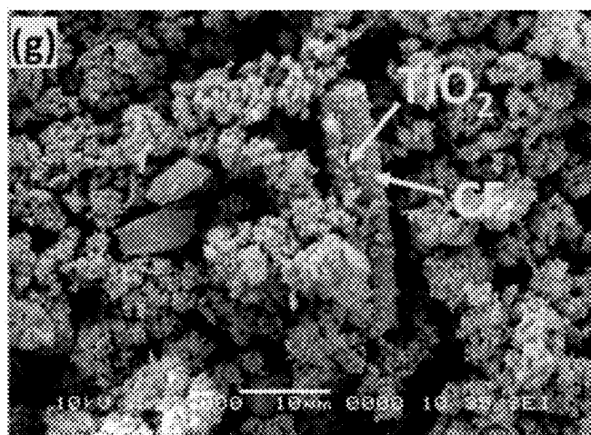
Fig. 7G - SEM images of 3CFs/TiO 2 -S
