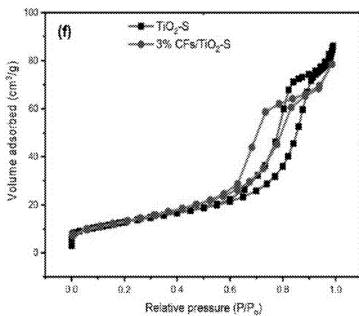
Fig. 11 - N 2 adsorption-desorption isotherms of TiO 2 -S and 3% CF/TiO 2 -S composite
