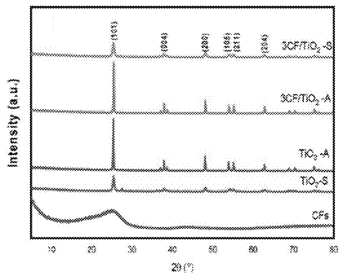
Fig. 4 - XRD patterns of CF, TiO_2 -A, TiO_2 -S, CF/TiO_2 -A, and CF/TiO_2 -S samples
