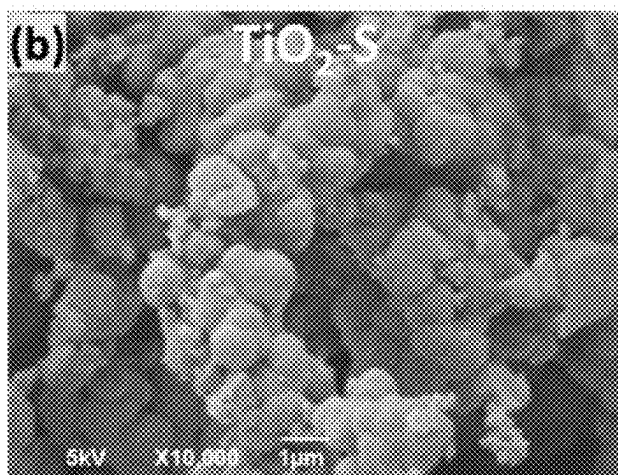
Fig. 7B - SEM images of \text{TiO}_2\text{-S}
