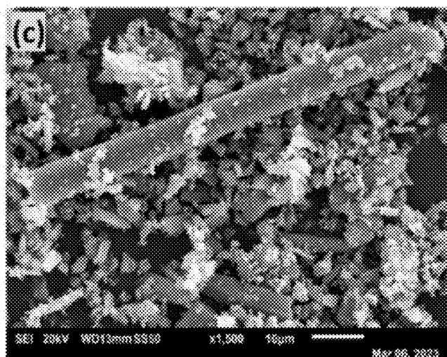
Fig. 7C - SEM images of CFs
