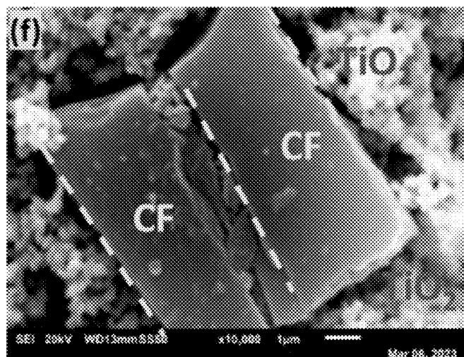
Fig. 7F - SEM images of 3CFs/TiO 2 -A
