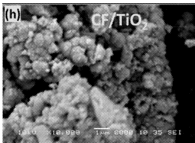
Fig. 7H - SEM images of 3CFs/TiO 2 -S
