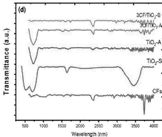
Fig. 6 - IR patterns of CF, TiO 2 -A, TiO 2 -S, CF/TiO 2 -A, and CF/TiO 2 -S samples
