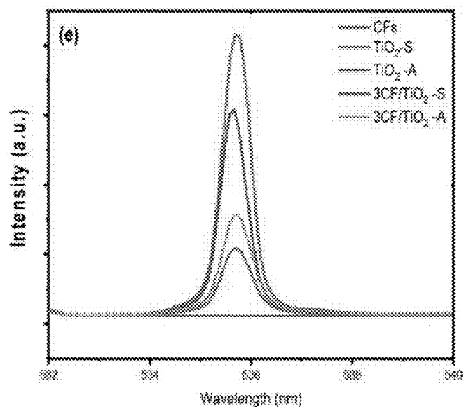
Fig. 10 - PL analysis of CF, TiO 2 -A, TiO 2 -S, and CF/TiO 2 -A and CF/TiO 2 -S composite samples
