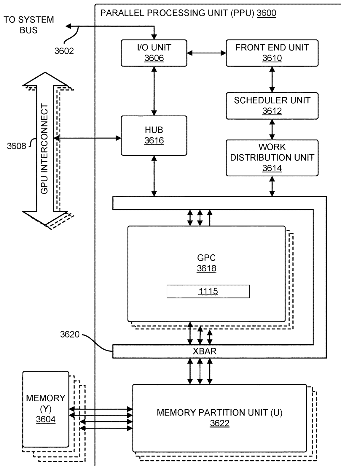
FIG. 36
