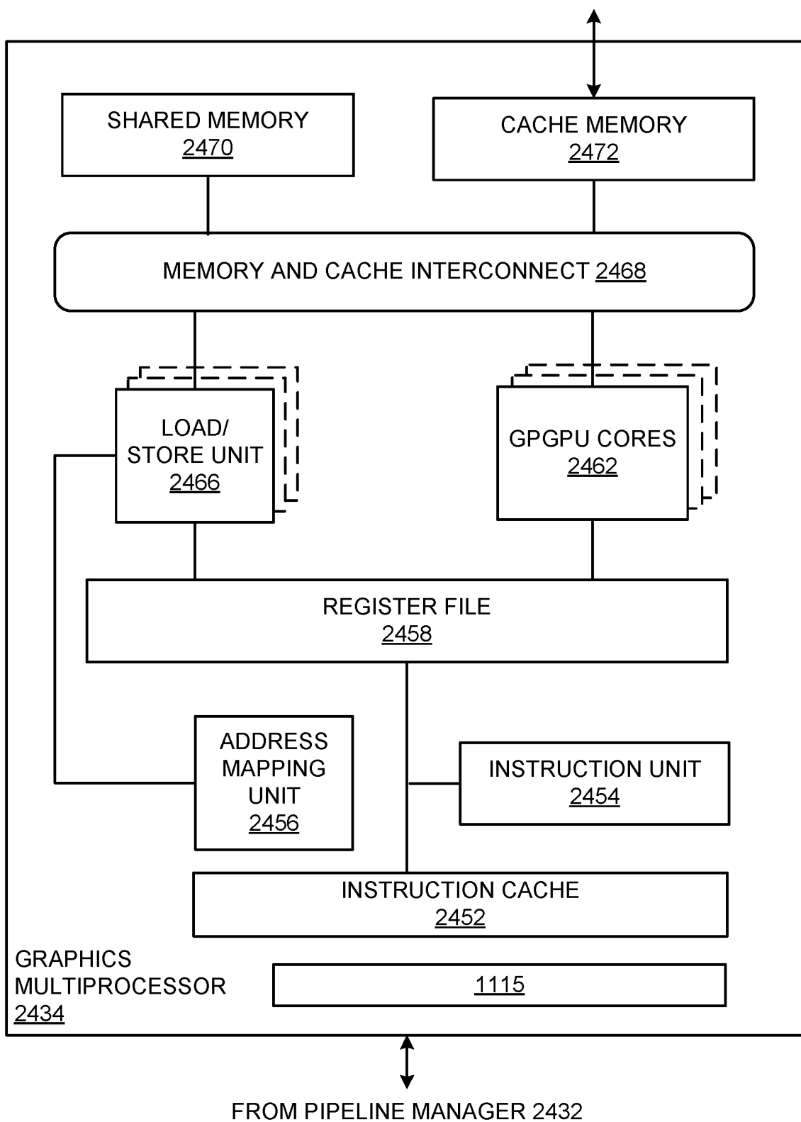
FIG. 24D
