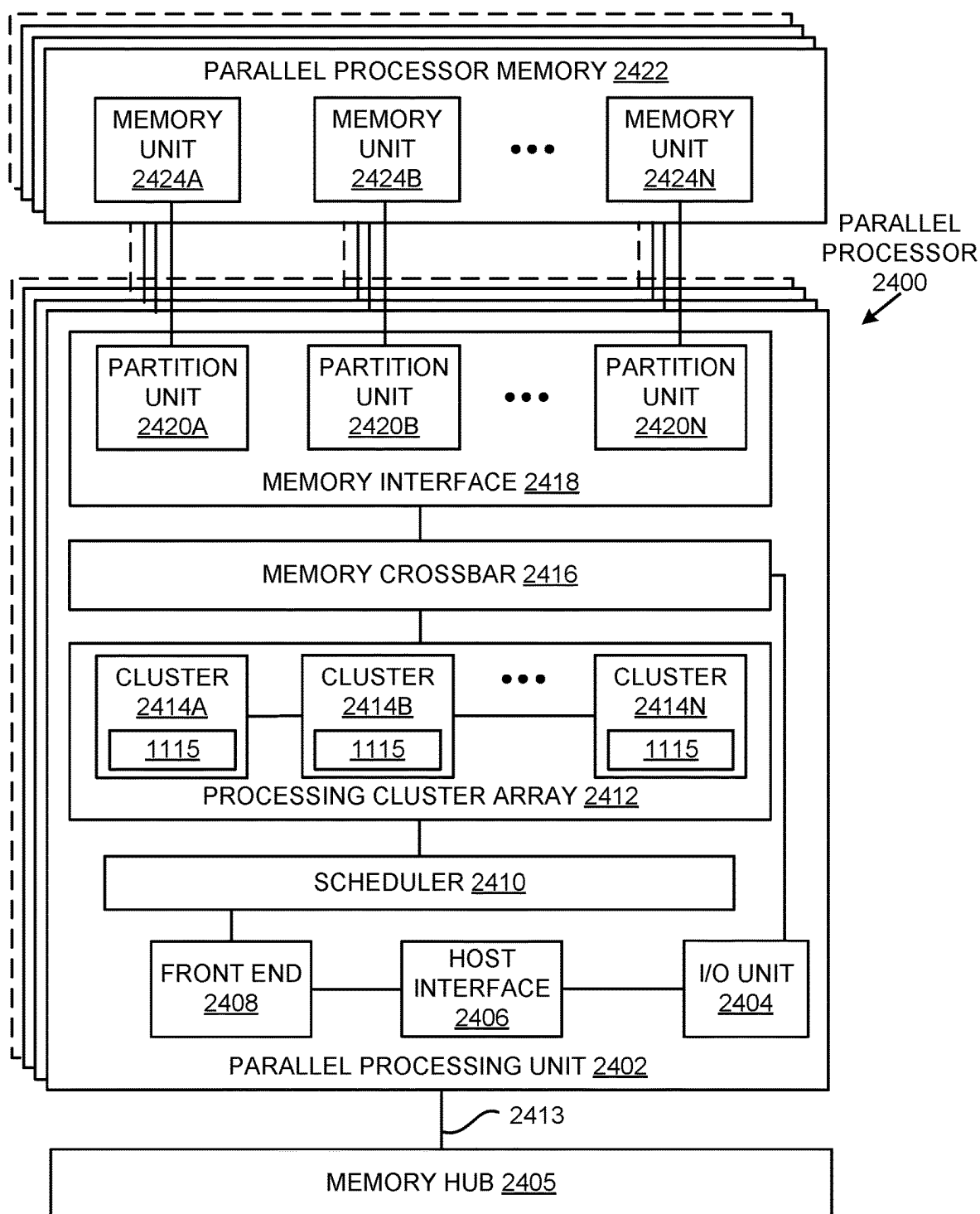
FIG. 24A
