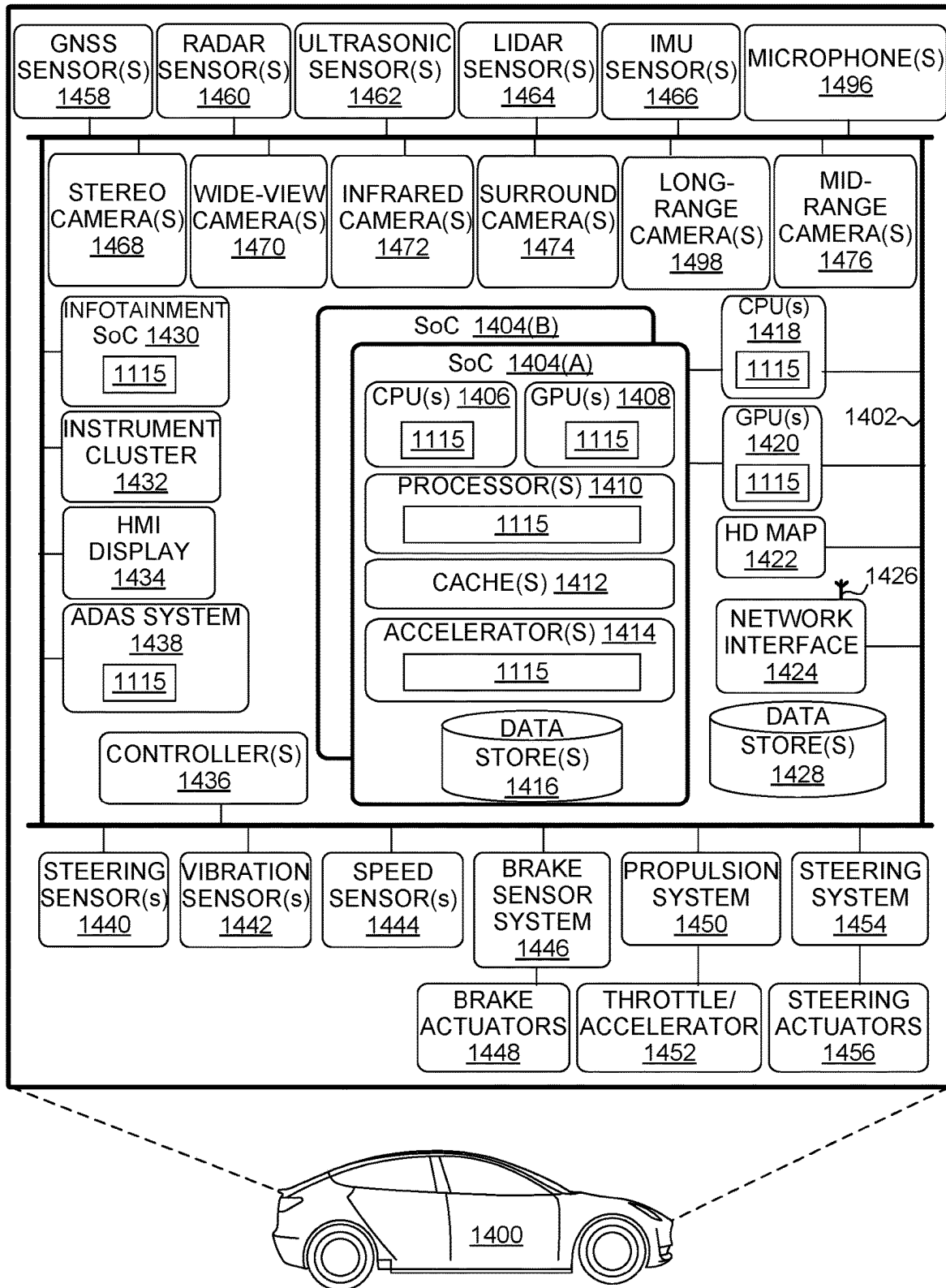
FIG. 14C
