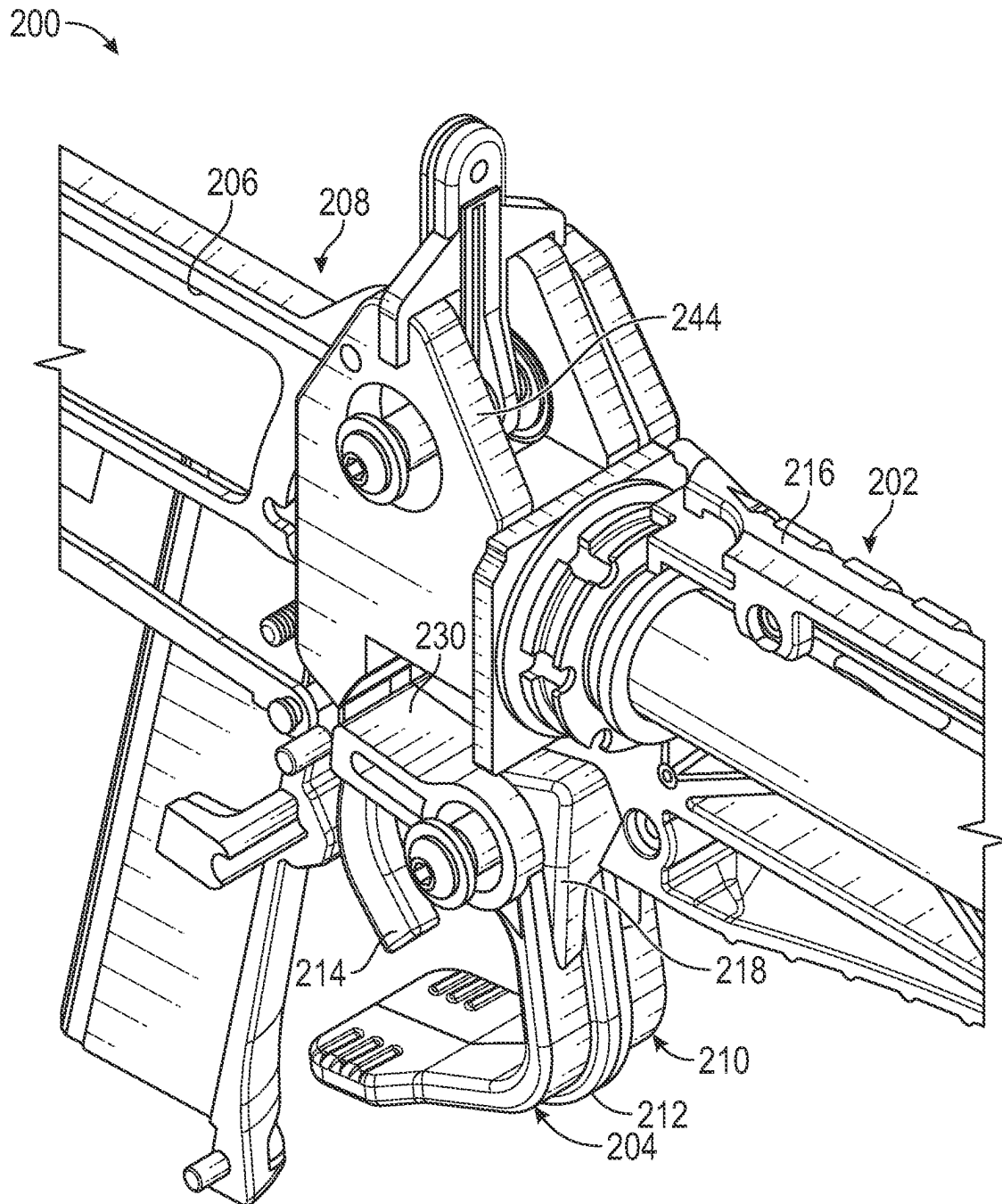
FIG. 13B
