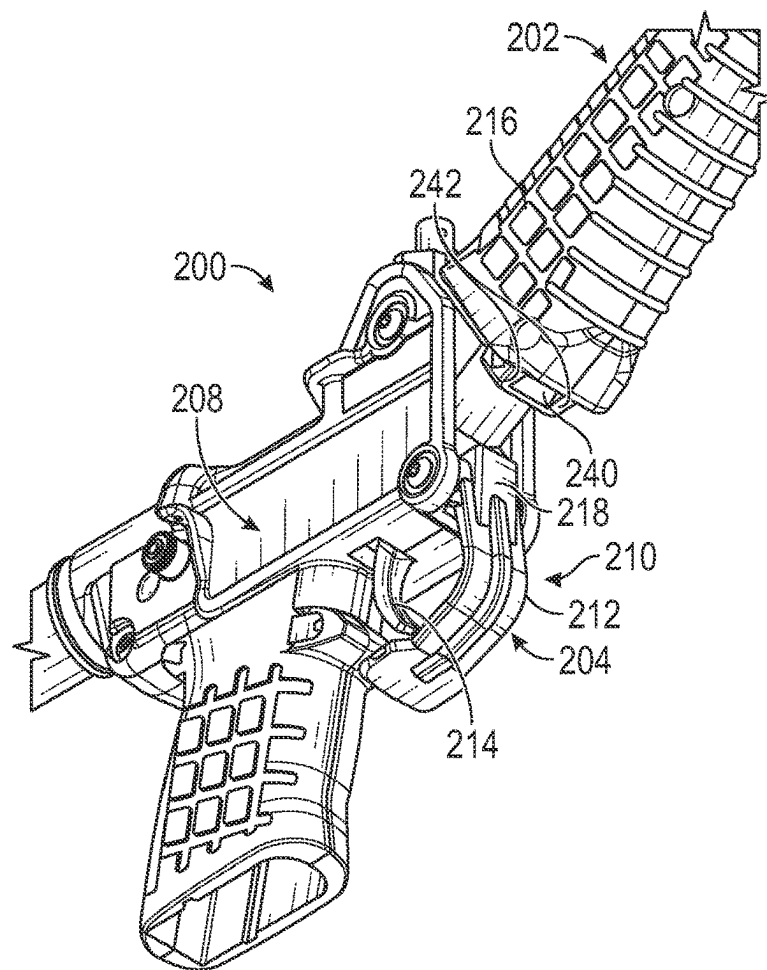
FIG. 14B
