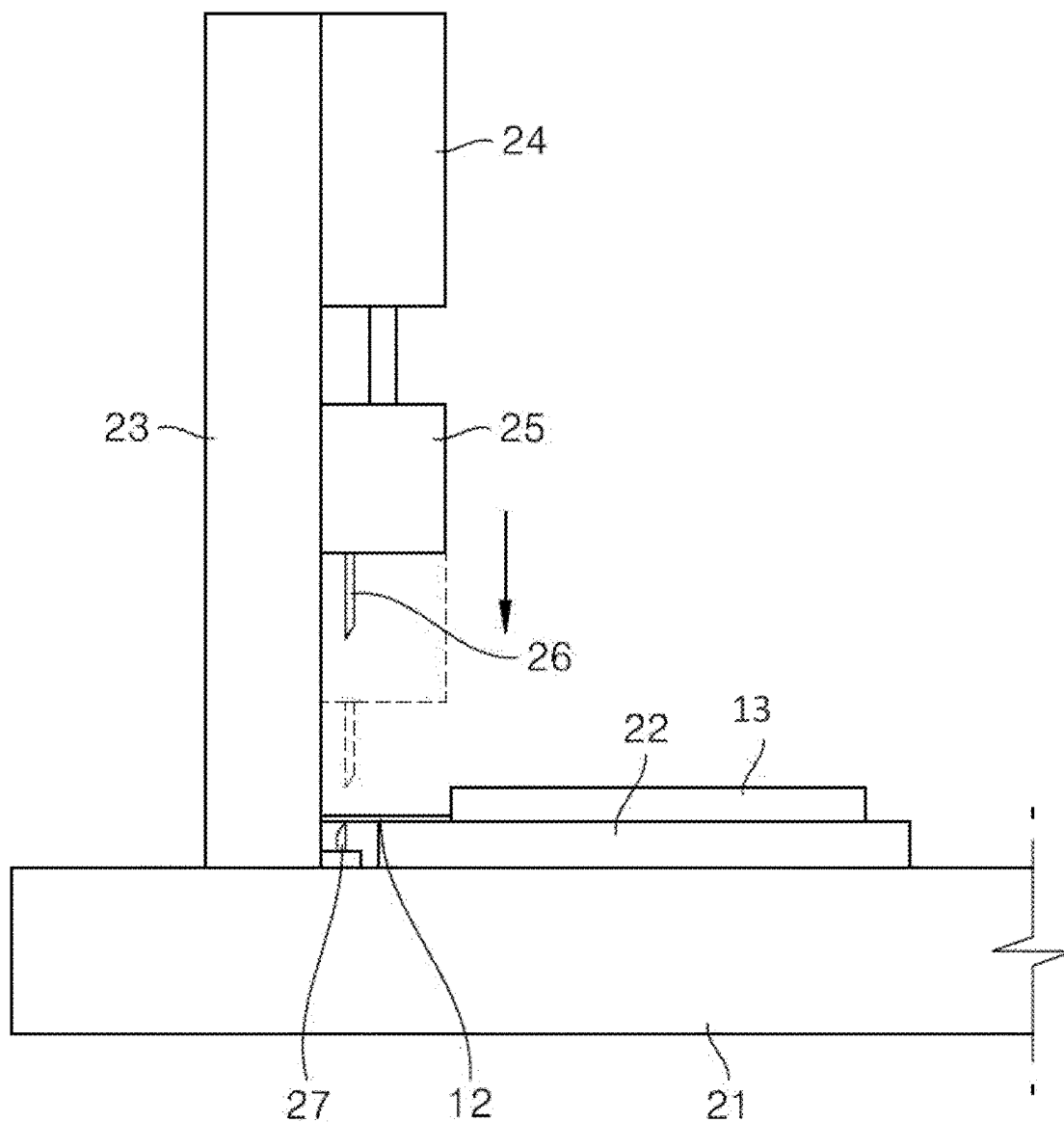
【FIG. 2】 (Conventional Art)
