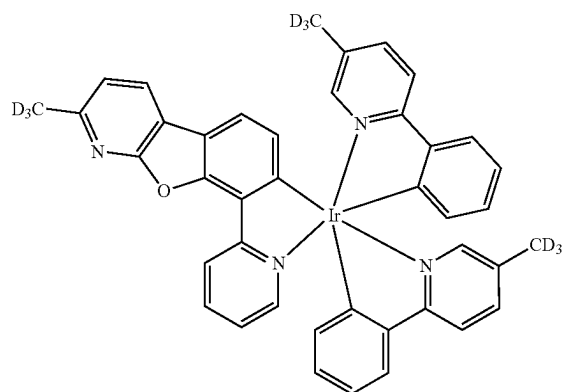
Ir(5mppy-d 3 ) 2 (mbfpypy-d 3 )
