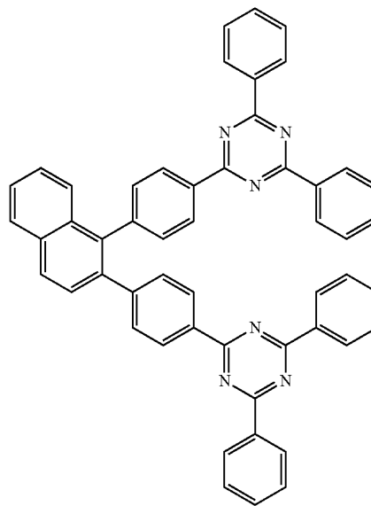
TznP2N
