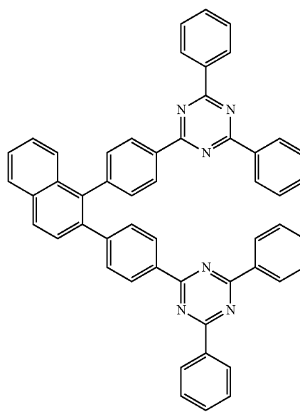
TznP2N
