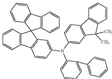
oFBiSF(2)
