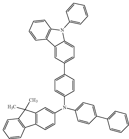
PCBBiF
