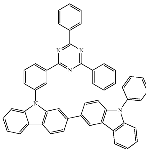
mPCCzPTzn-02
