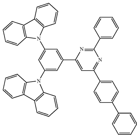
6BP-4Cz2PPm
