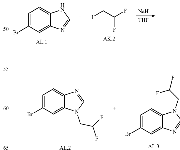
Scheme AL
