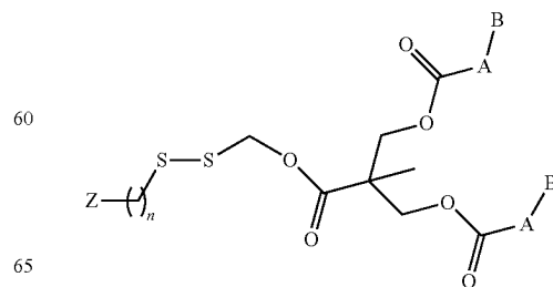
Formula Ic
