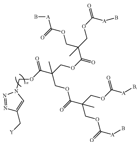
Formula Ic
