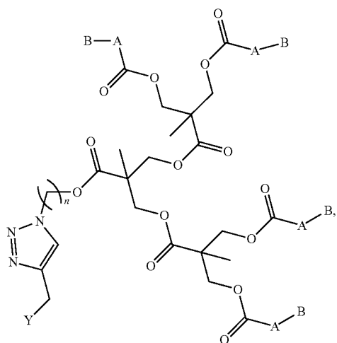
Formula Ic
