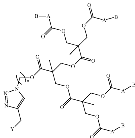
Formula Ic
