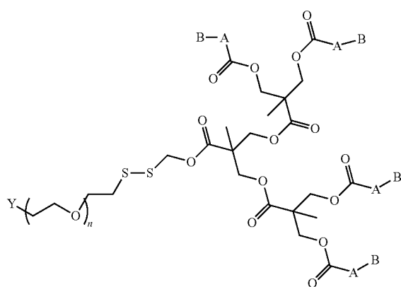
Formula Ij
