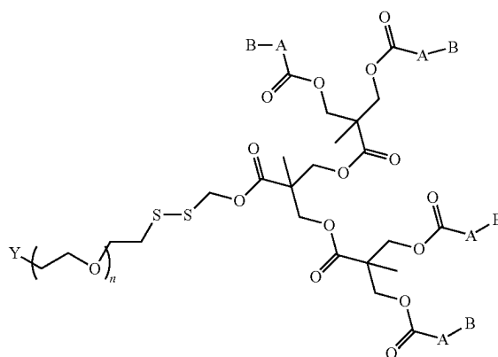
Formula Ij
