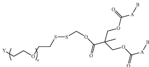
Formula Ij
