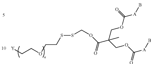
Formula Ij
