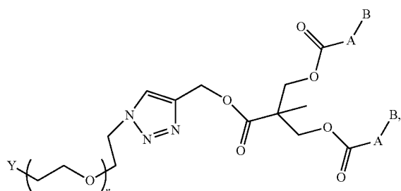
Formula Ic
