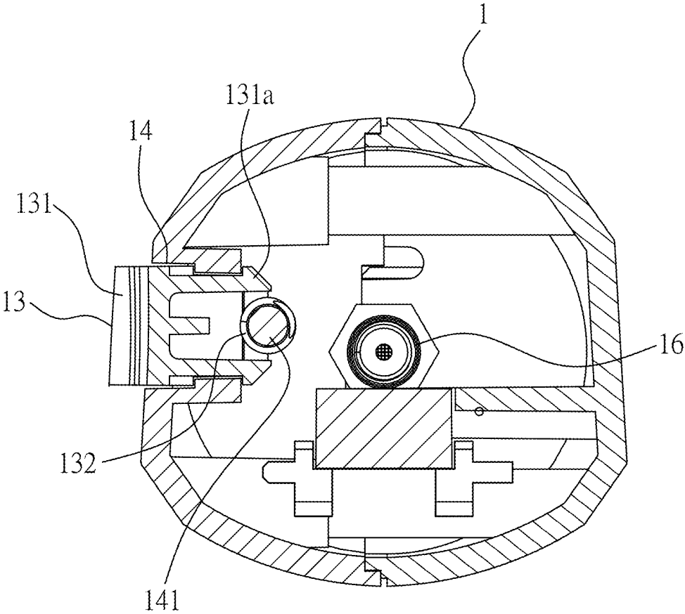
A-A FIG. 5
