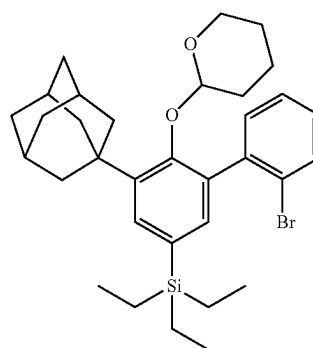
(5-(1-adamantyl)-2'-bromo-6-((tetrahydro-2H-pyran-2-yl)oxy)-[1,1'-biphenyl]-3-yl)triethylsilane
