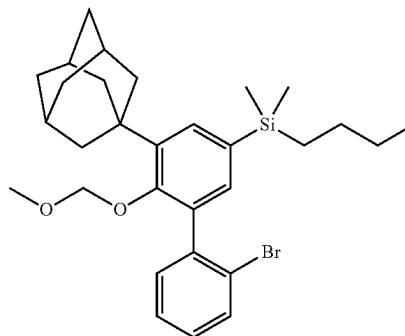
(5-(1-adamantyl)-2'-bromo-6-(methoxymethoxy)-[1,1'-biphenyl]-3-yl)(butyl)dimethylsilane
