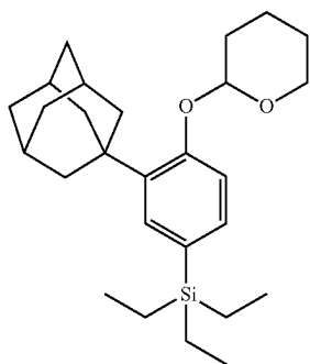
(3-(1-adamantyl)-4-((tetrahydro-2H-pyran-2-yl)oxy)phenyl)triethylsilane
