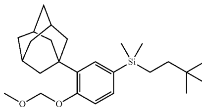
(3-(1-adamantyl)-4-(methoxymethoxy)phenyl)(3,3-dimethylbutyl)dimethylsilane
