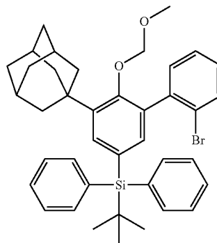
(5-(1-adamantyl)-2'-bromo-6-(methoxymethoxy)-[1,1'-biphenyl]-3-yl)(tert-butyl)diphenylsilane
