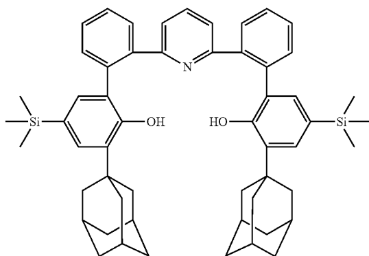
2',2'''-(Pyridine-2,6-diyl)bis(3-(1-adamantyl)-5-(trimethylsilyl)-[1,1'-biphenyl]-2-ol)
