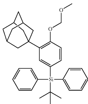
(3-(1-adamantyl)-4-(methoxymethoxy)phenyl)(tert-butyl)diphenylsilane
