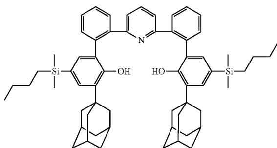
2',2'''-(pyridine-2,6-diyl)bis(3-(1-adamantyl)-5-(butyldimethylsilyl)-[1,1'-biphenyl]-2-ol)
