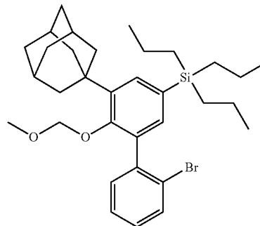
(5-(1-adamantyl)-2'-bromo-6-(methoxymethoxy)-[1,1'-biphenyl]-3-yl)triethylsilane
