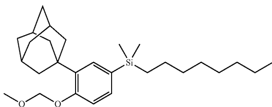
(3-(1-adamantyl)-4-(methoxymethoxy)phenyl)(octyl)dimethylsilane
