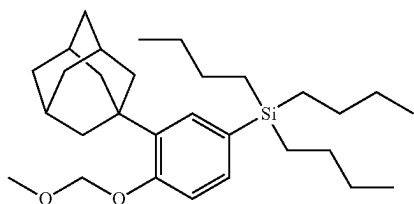
(3-(1-adamantyl)-4-(methoxymethoxy)phenyl)tributylsilane
