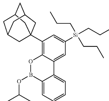
(4-(1-adamantyl)-6-isopropoxy-benzo[c][1,2]benzoxaborinin-2-yl)triethylsilane
