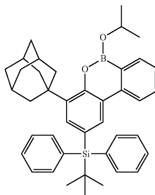
(4-(1-adamantyl)-6-isopropoxy-benzo[c][1,2]benzoxaborinin-2-yl)(tert-butyl)diphenylsilane
