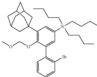
(5-(1-adamantyl)-2'-bromo-6-(methoxymethoxy)-[1,1'-biphenyl]-3-yl)tributylsilane
