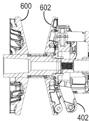
SECTION A-A FIG. 24I
