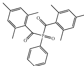
OMNIRAD 819
