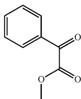
OMNIRAD MBF
