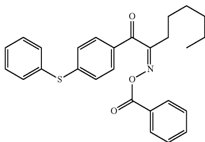
IRGACURE® OXE-01
