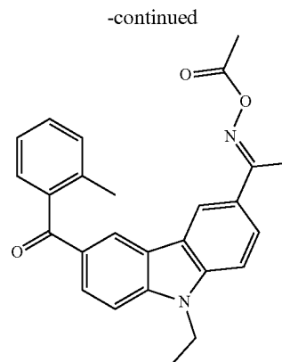
IRGACURE® OXE-02
