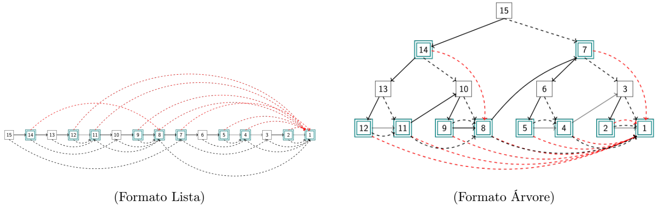
Figura 9: Representação da IARASS
