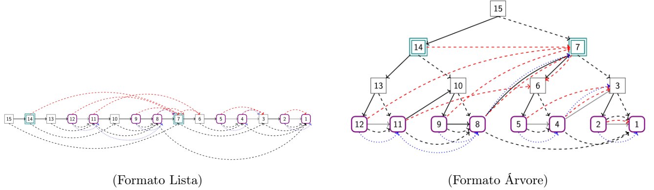
Figura 8: Representação da Dense Advanced Myers List
