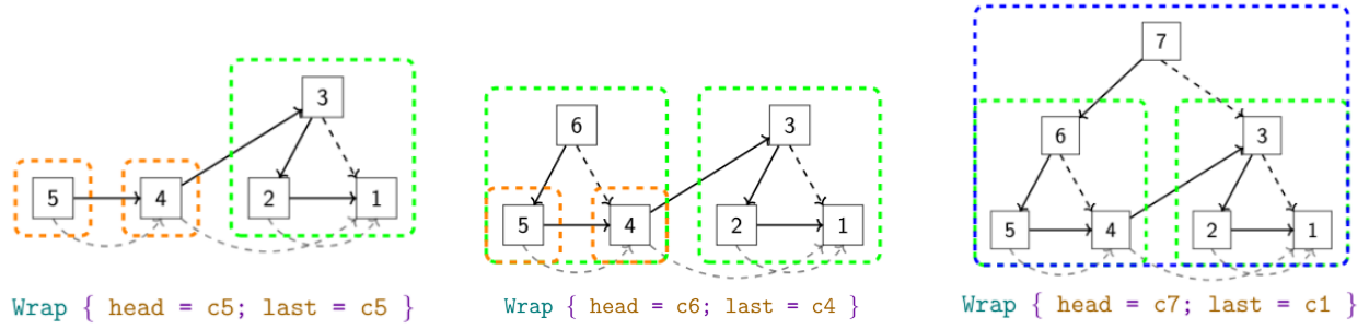
Figura 5: wrap durante o cons na Improved Myers List
