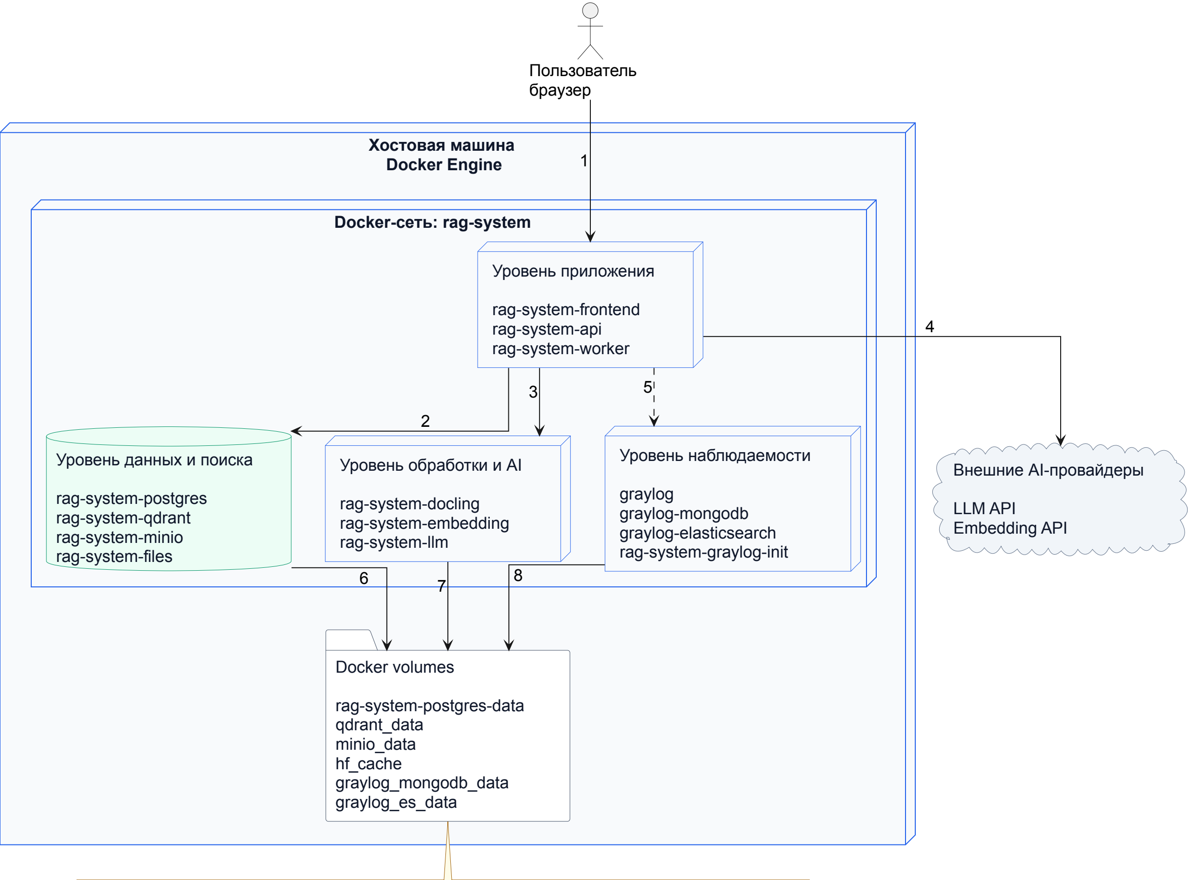
Диаграмма развёртывания RAG-системы
