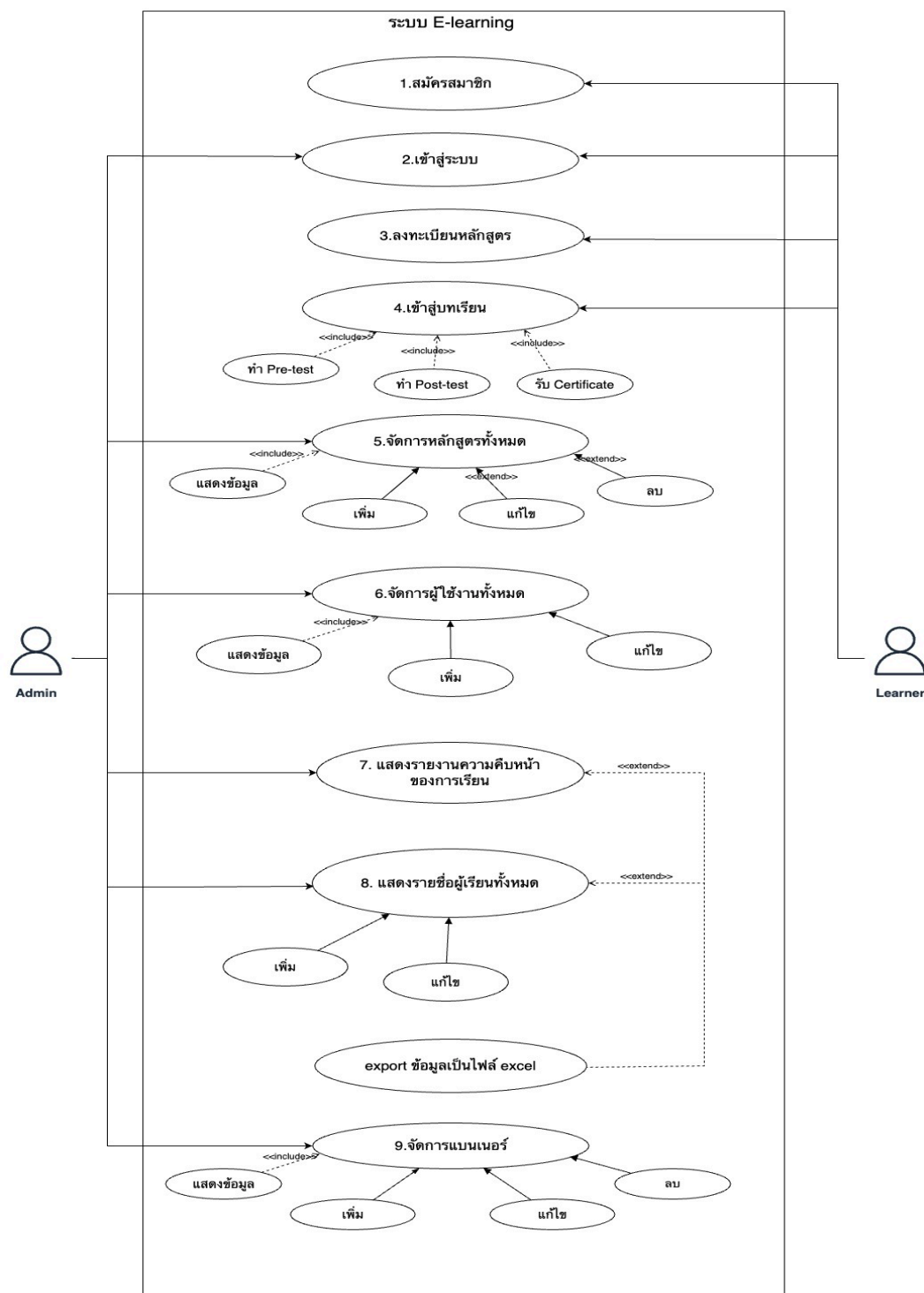
รูปที่ 3.2 Use Case Diagram ระบบการเรียนรู้ผ่านสื่ออิเล็กทรอนิกส์
