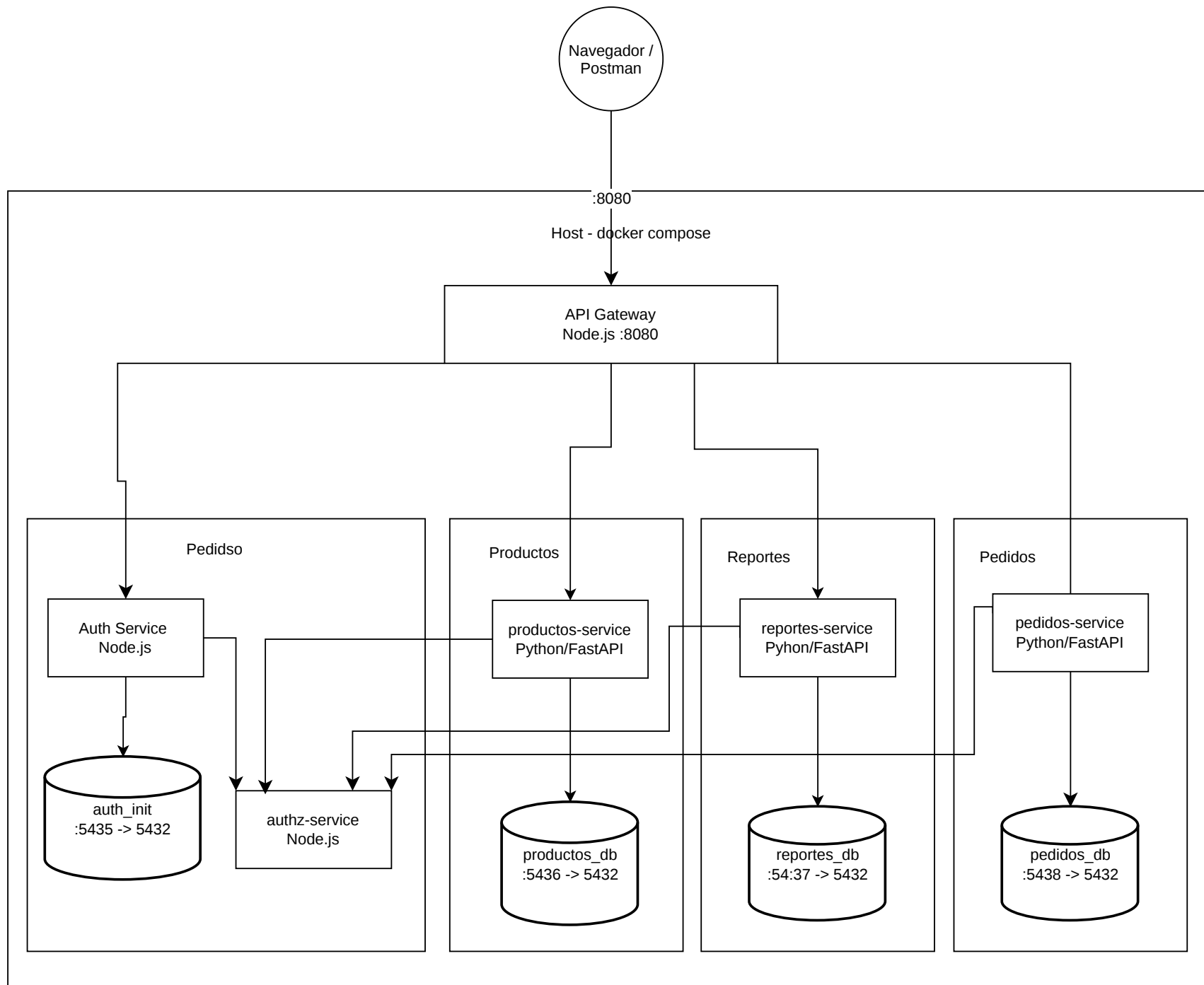
Diagrama de despliegue
