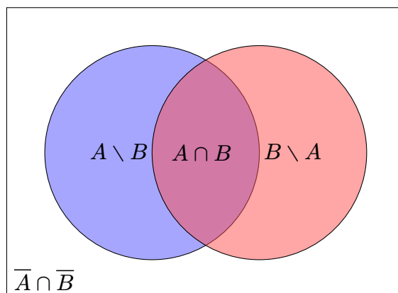
Venn-Diagramm
