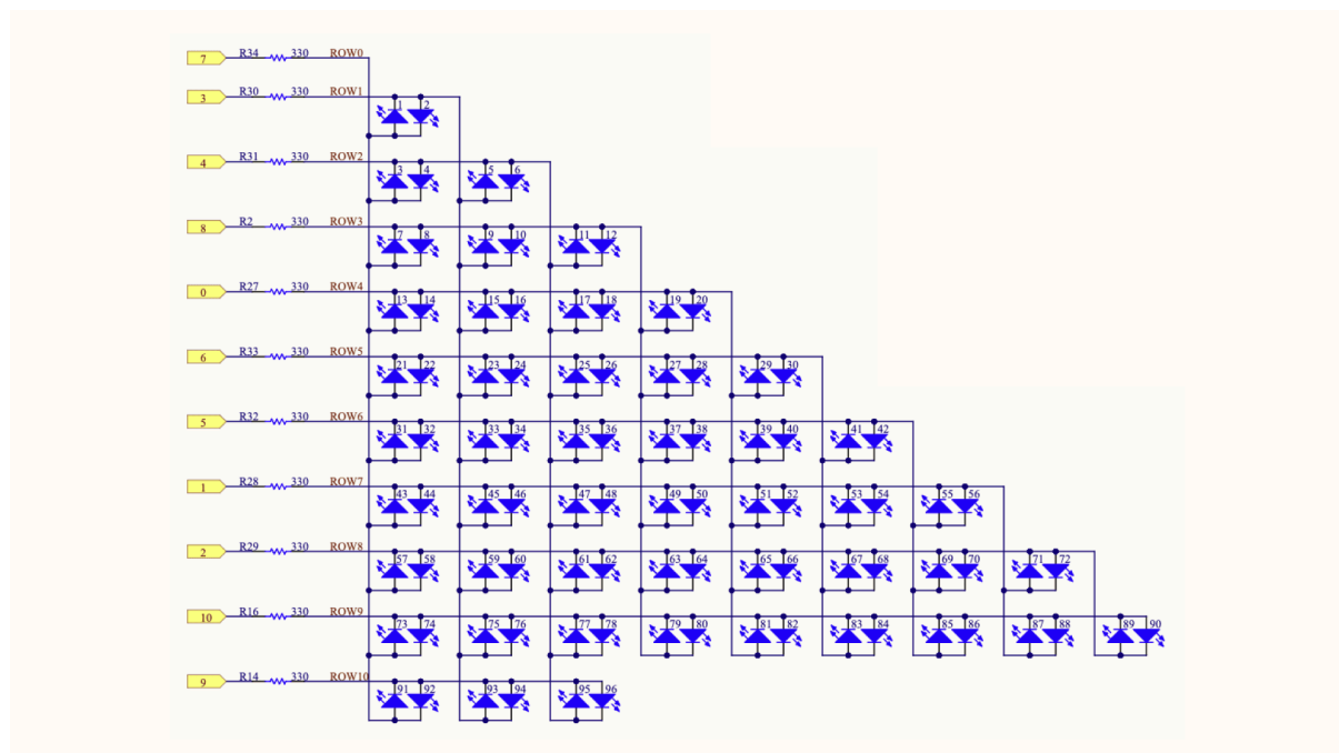
LED矩阵示意图
