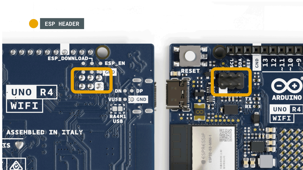
ESP 针脚
