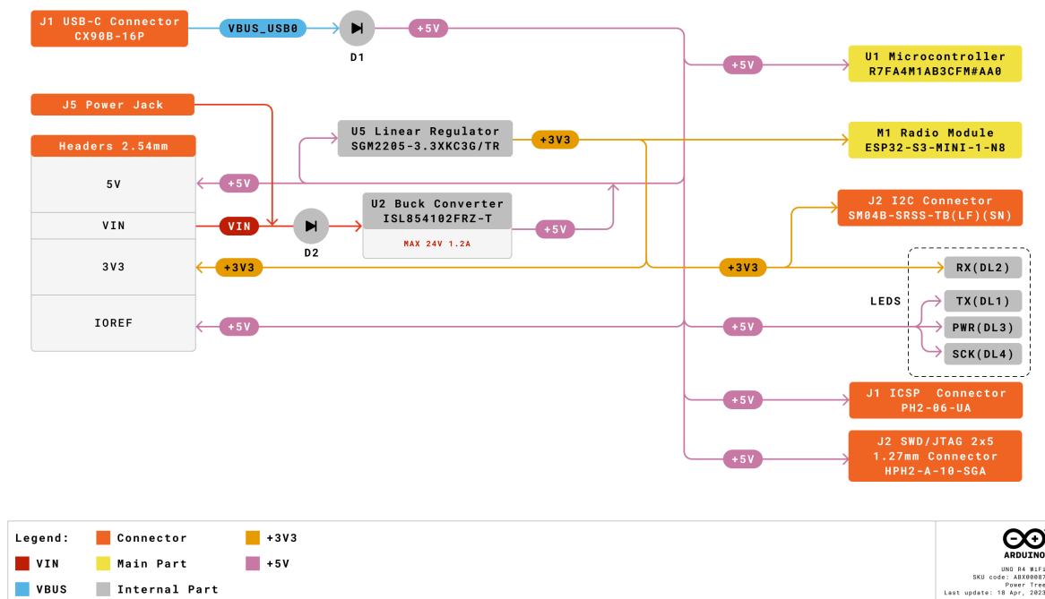
Arduino UNO R4 WiFi电源树
