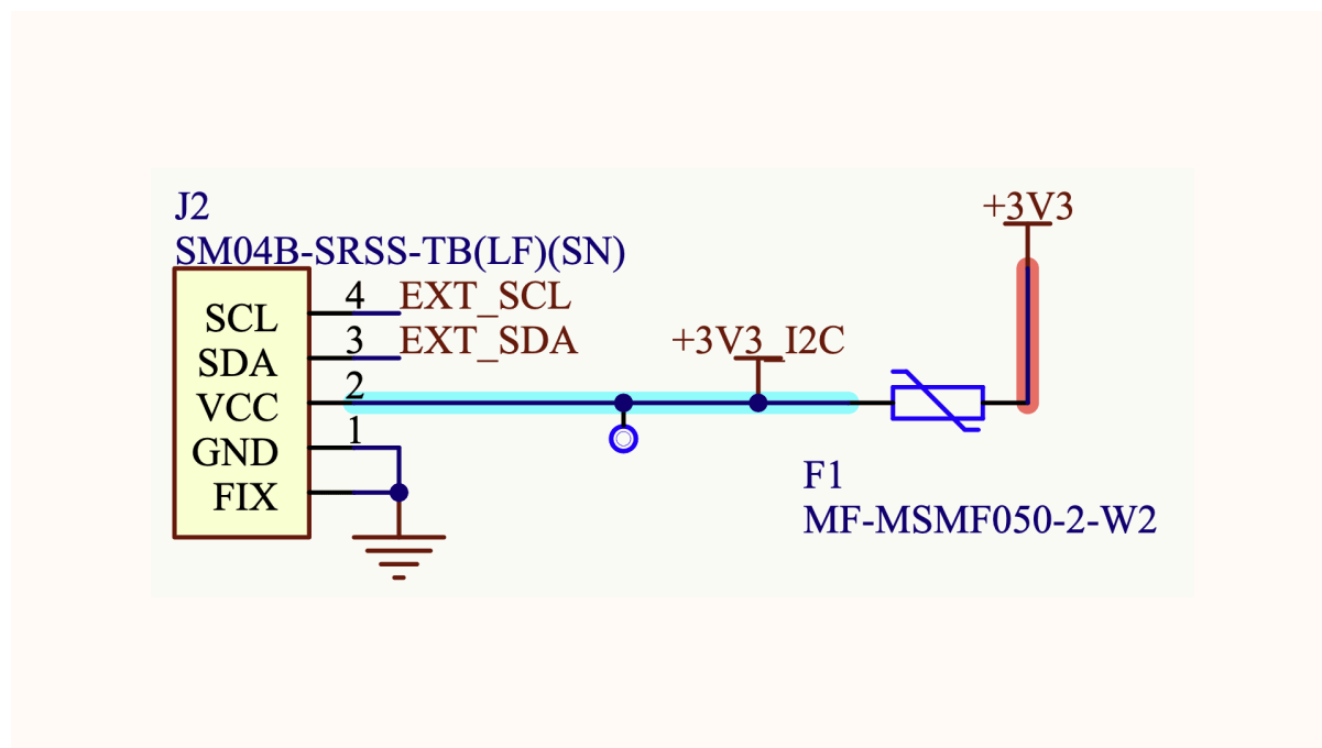
I2C连接器
