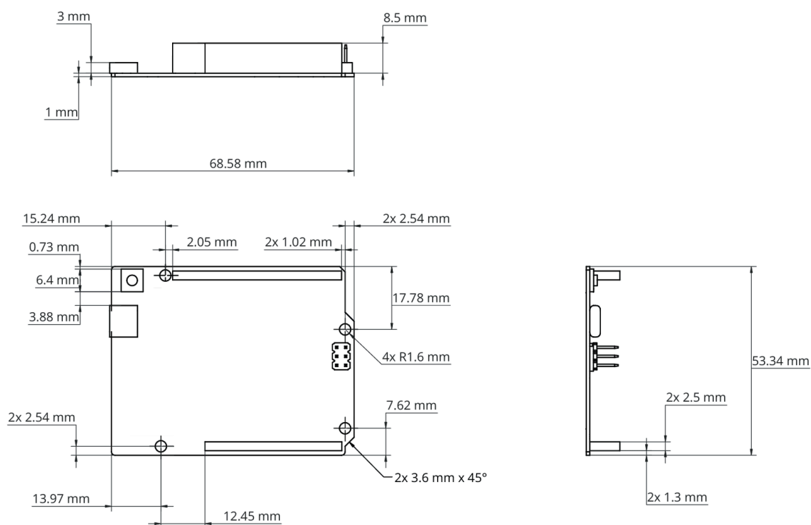
Arduino UNO R4 WiFi 的顶部机械视图
