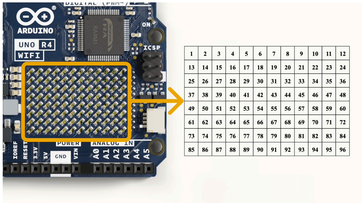
LED矩阵编号映射
