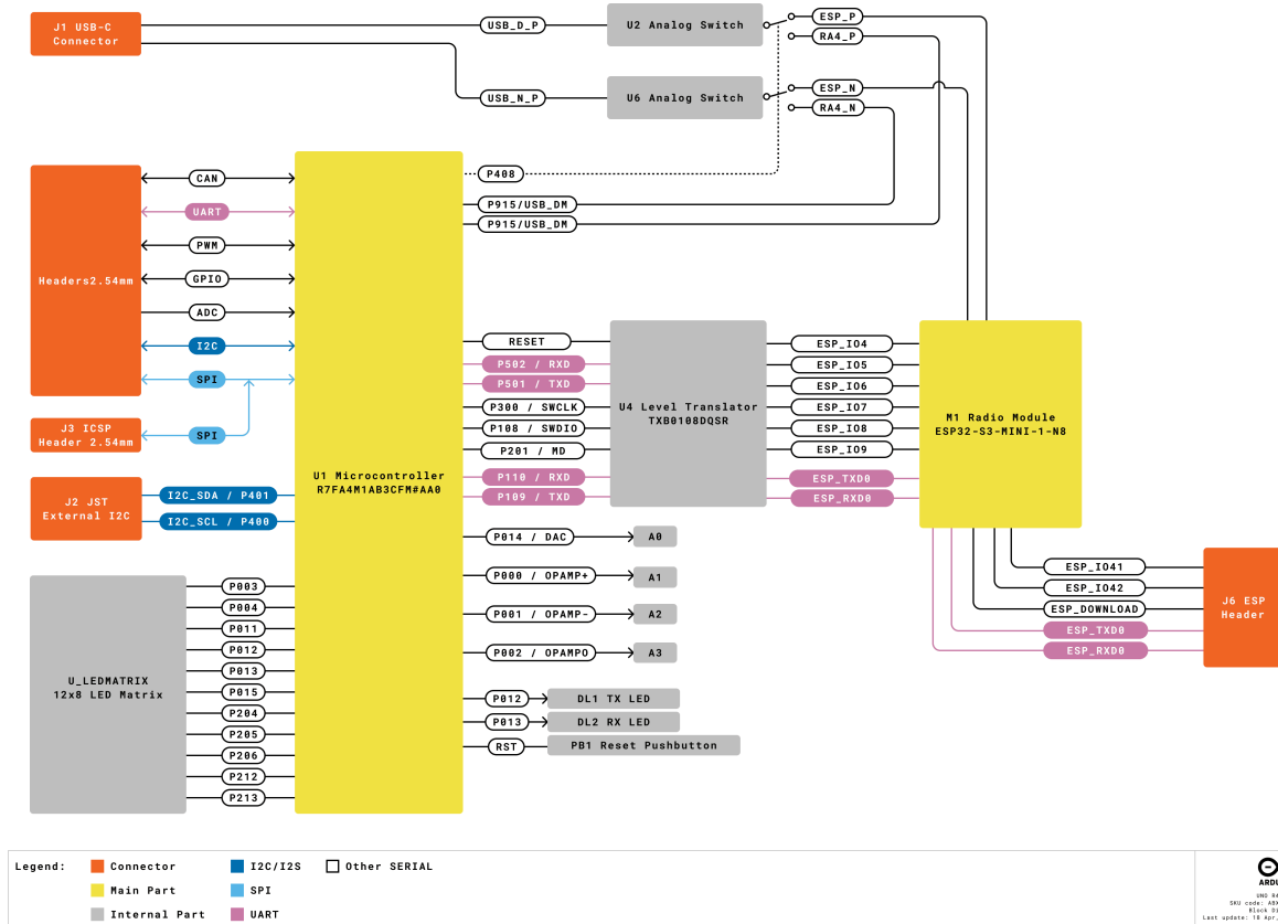
Arduino UNO R4 WiFi 框图
