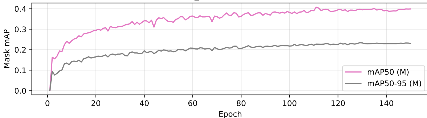
YOLO26n_seg Mask Validation mAP
