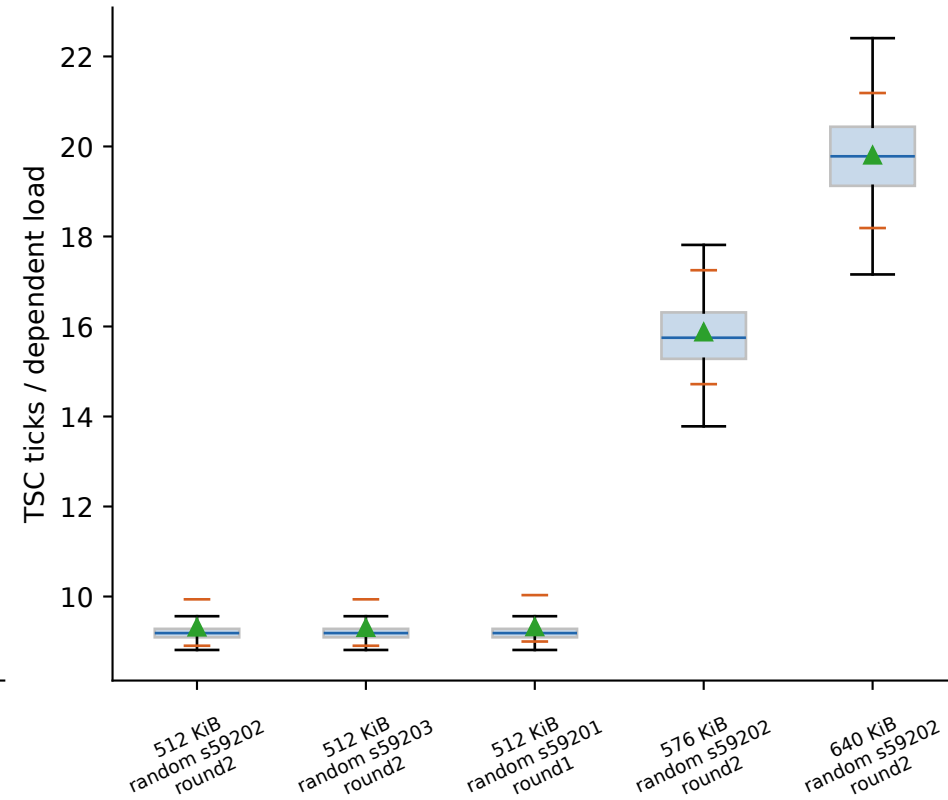
skylark: L2
