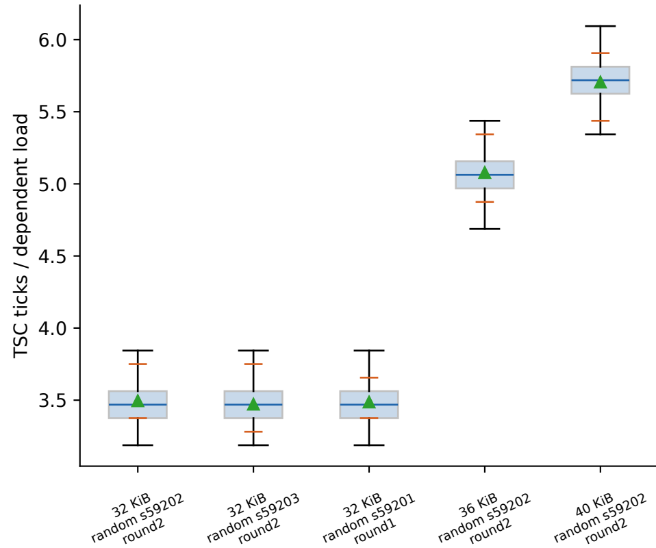
skylark: L1D
