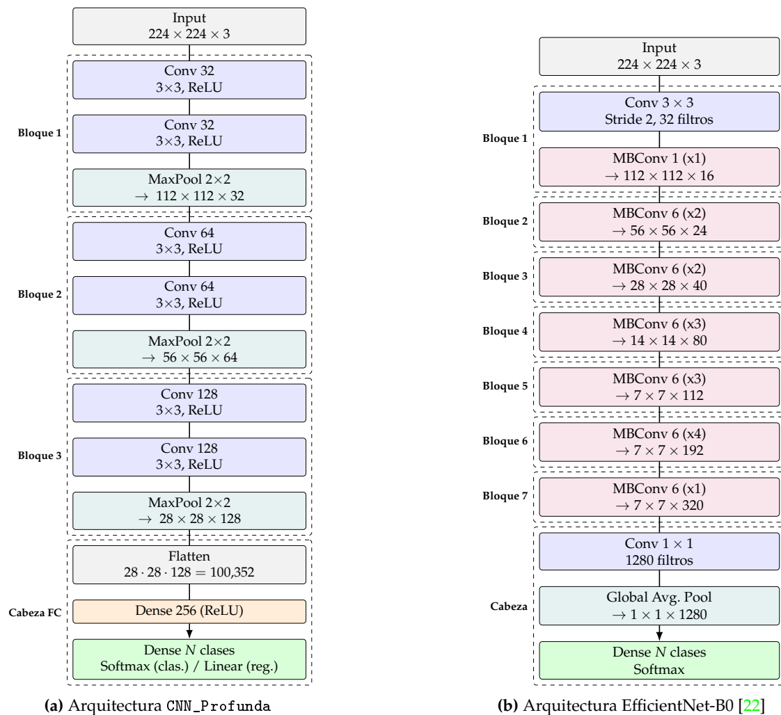
Figura 4.4: Comparación de arquitecturas de redes neuronales convolucionales. (a) Arquitectura de una CNN profunda tradicional. (b) Arquitectura de EfficientNet-B0.
