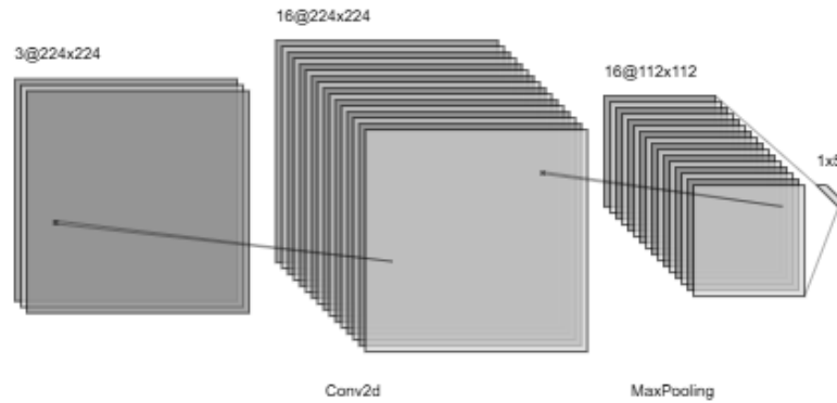
Figura 4.1: Esquema AlexNet-style de la CNN simple (línea base)
