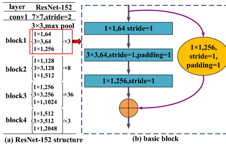
Figura 4.3: Esquema de ResNet152 [21]
