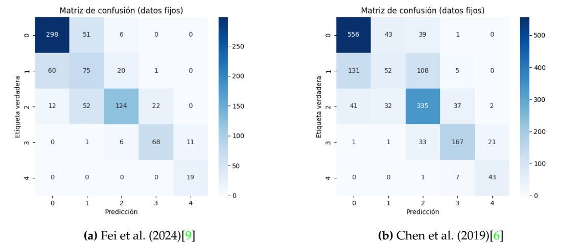
Figura 3.5: Matrices de confusión agregadas en la clasificación multiclase KL 0–4 con los mejores modelos de Fei et al. (2024) y Chen et al. (2019). Se observa que los aciertos predominan en la diagonal y las confusiones se concentran entre clases vecinas, especialmente en las clase 1
