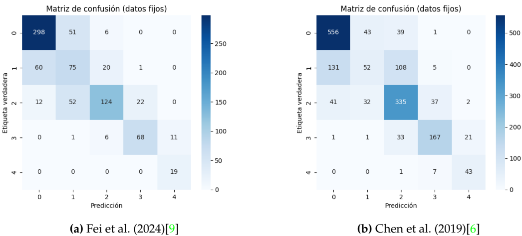
Figura 3.5: Matrices de confusión agregadas en la clasificación multiclase KL 0–4 con los mejores modelos de Fei et al. (2024) y Chen et al. (2019). Se observa que los aciertos predominan en la diagonal y las confusiones se concentran entre clases vecinas, especialmente en las clase 1
