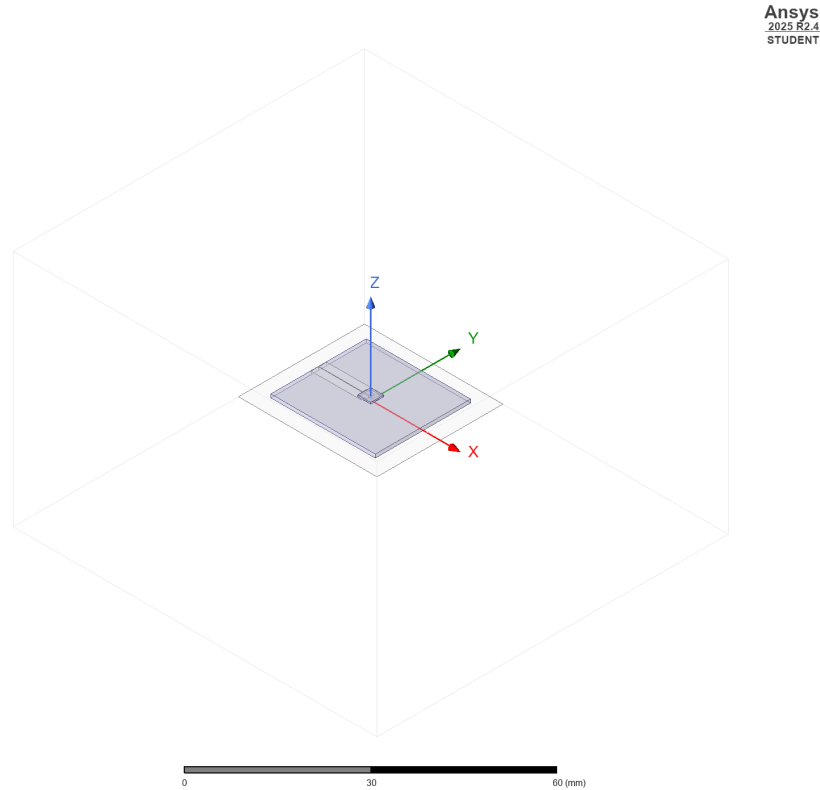
Figura 4: Vista isométrica do modelo, exportada diretamente do Ansys HFSS ( export_model_picture ).
