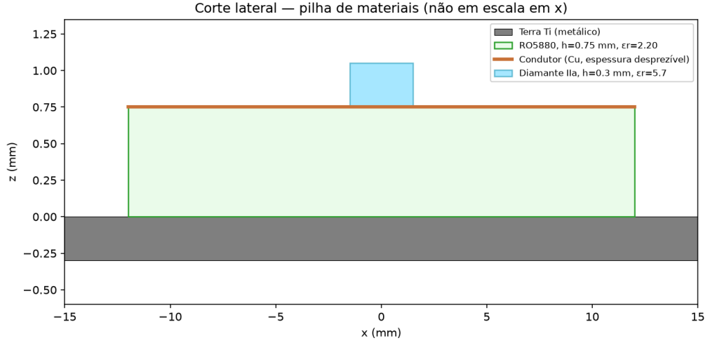
Figura 3: Corte lateral da pilha de materiais (terra de Ti, substrato RO5880, condutor, diamante). Escala vertical exagerada para clareza.
