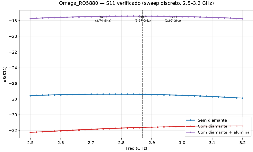
Figura 8: S_{11} verificado (varredura discreta) na banda de interesse, para as três configurações, com as transições Zeeman marcadas.
