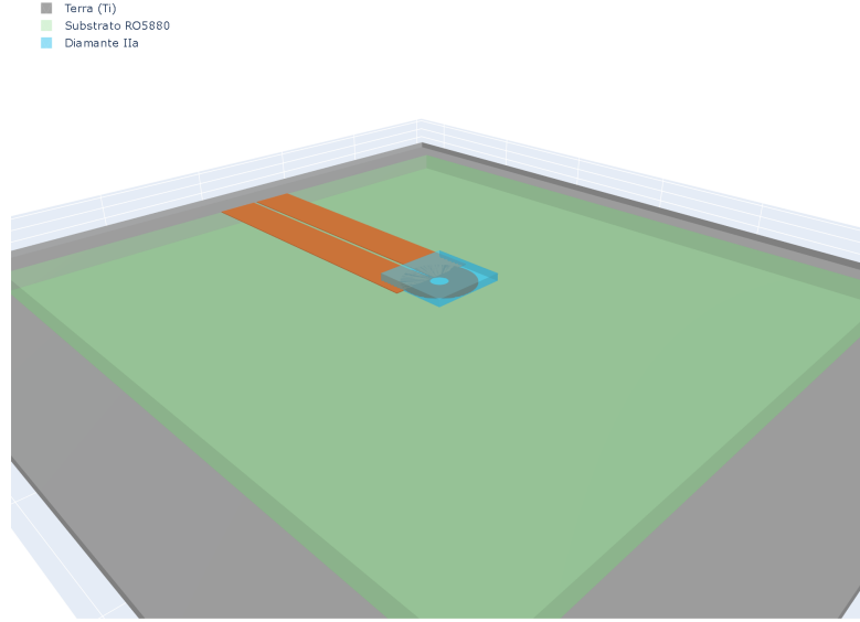
Ressorador ômega — vista 3D completa
