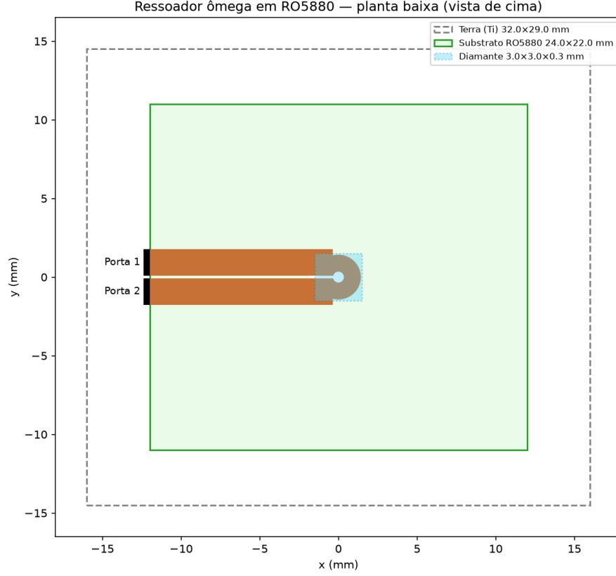
Figura 1: Planta baixa esquemática do ressoador (terra, substrato, condutor, diamante e portas), com as dimensões finais.
