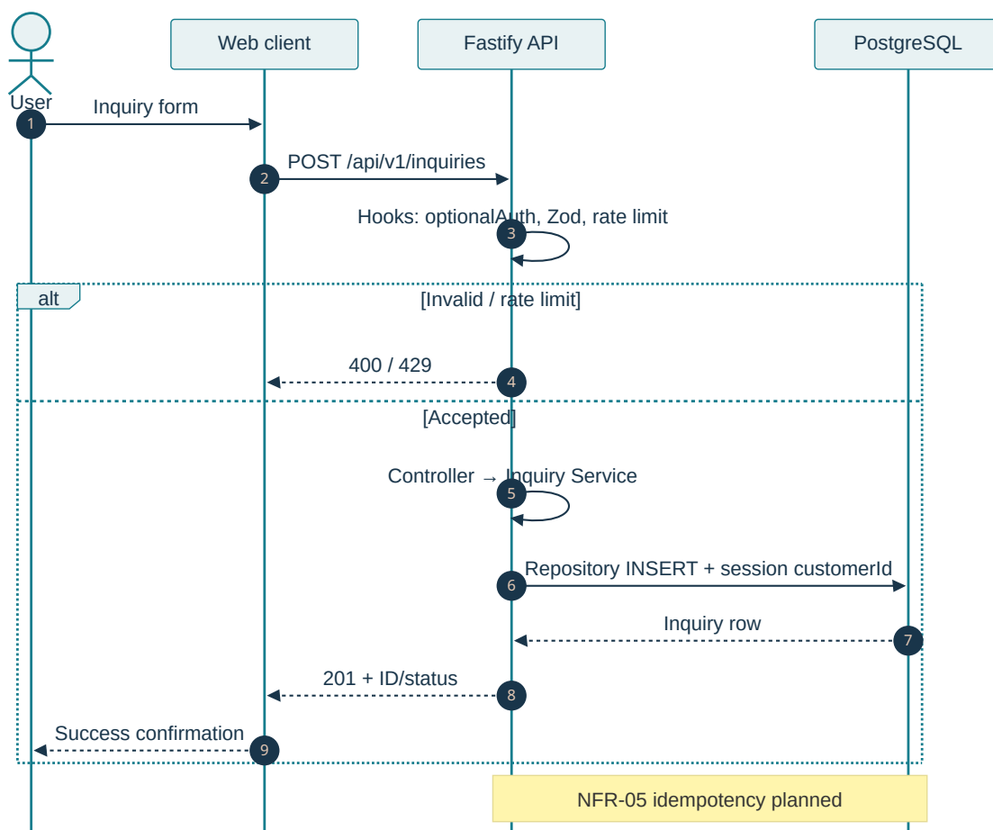
Зураг 4: C4-D01 — Inquiry Runtime
