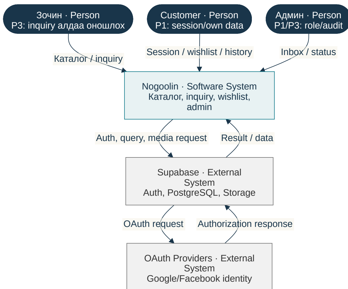
Зураг 1: C4-01 — Nogoolin System Context
