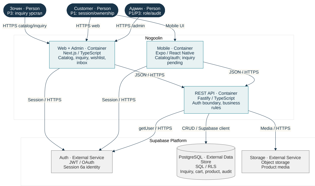
Зураг 8: UE-4 After — Nogoolin Container View
