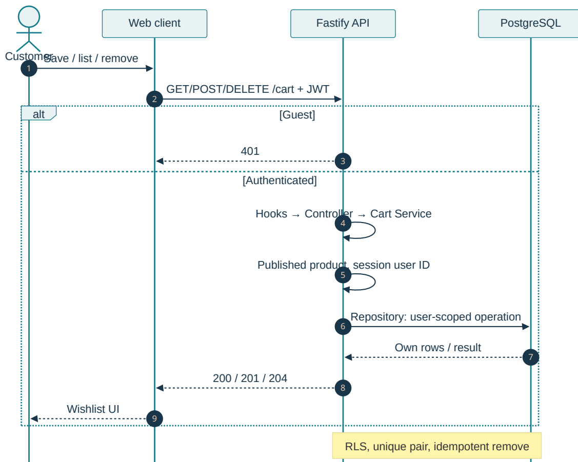
Зураг 5: C4-D02 — Wishlist Runtime
