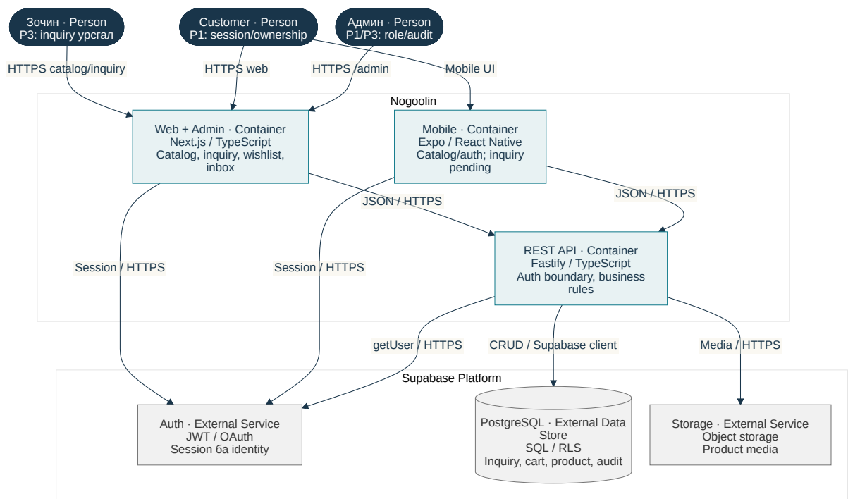
Зураг 2: C4-02 — Nogoolin Container View
