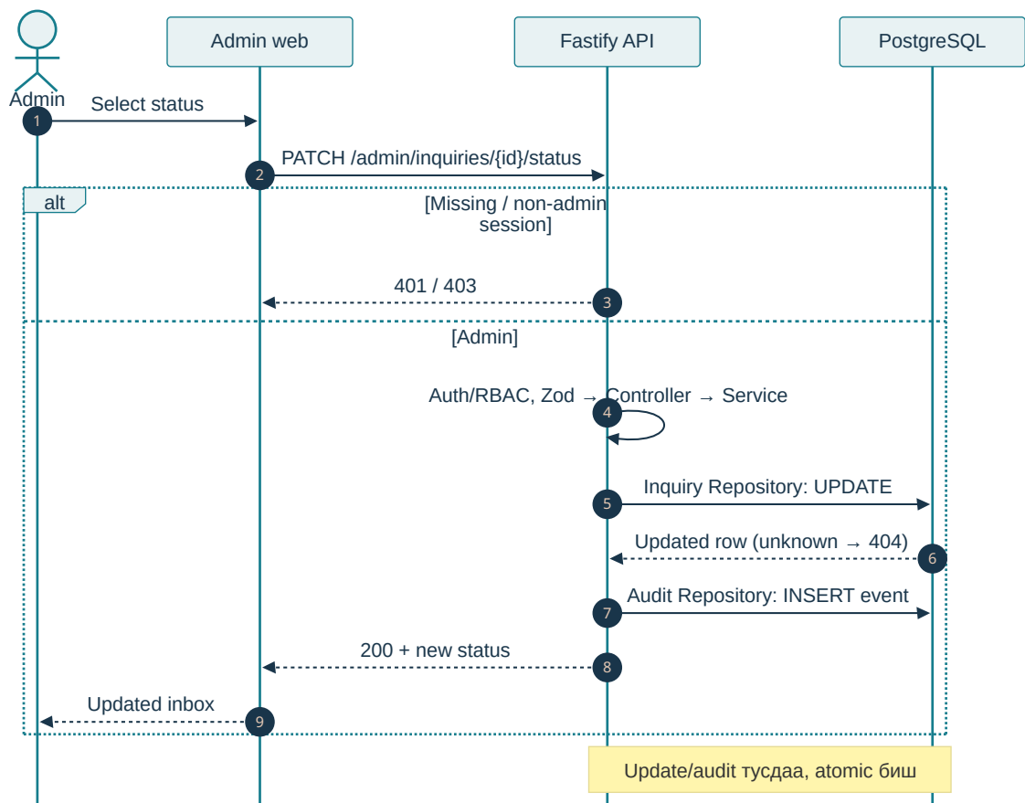
Зураг 6: C4-D03 — Admin Inquiry Runtime
