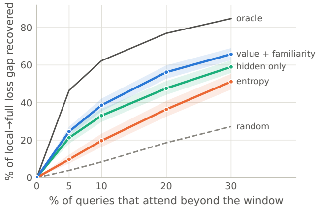
(a) Pythia-1.4B · 1k context · window 256 · 5 splits
