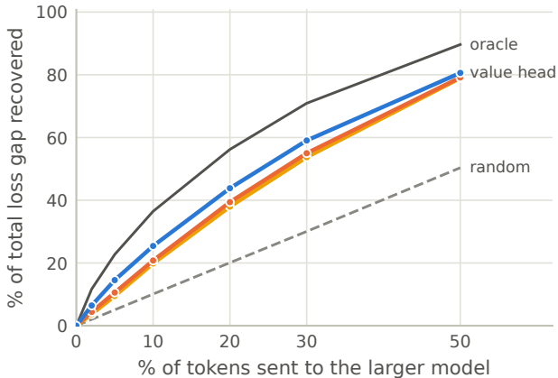
(a) compute: Pythia-160M \rightarrow 1.4B
