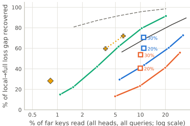
Qwen2.5-1.5B · 4k context · window 1024
