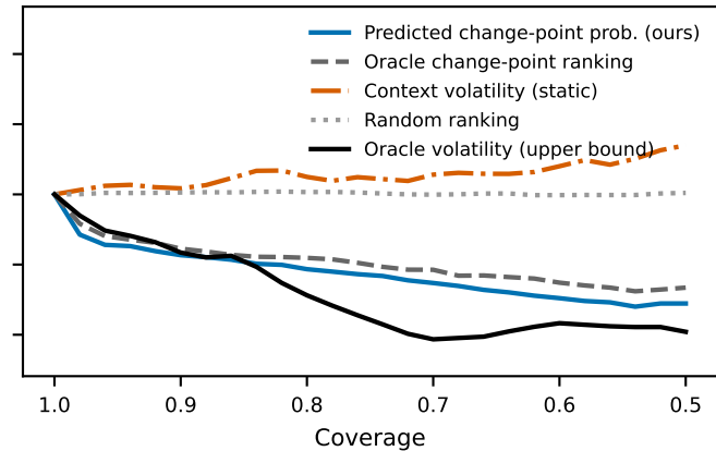
ETTM1
