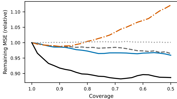
ETTh1
