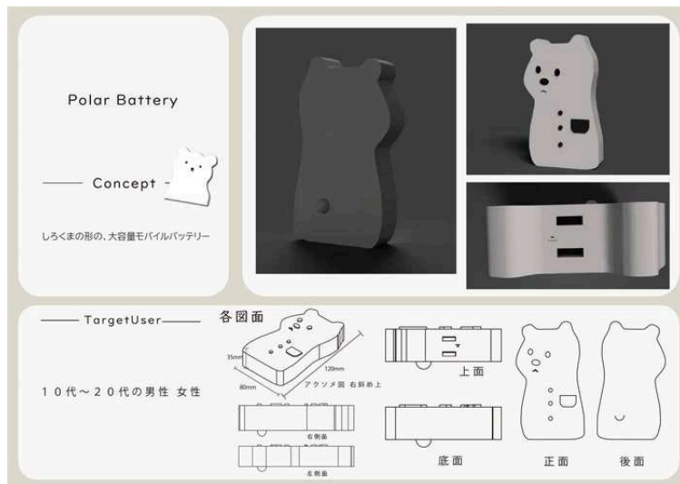
コンセプト・レンダリング・各図面
