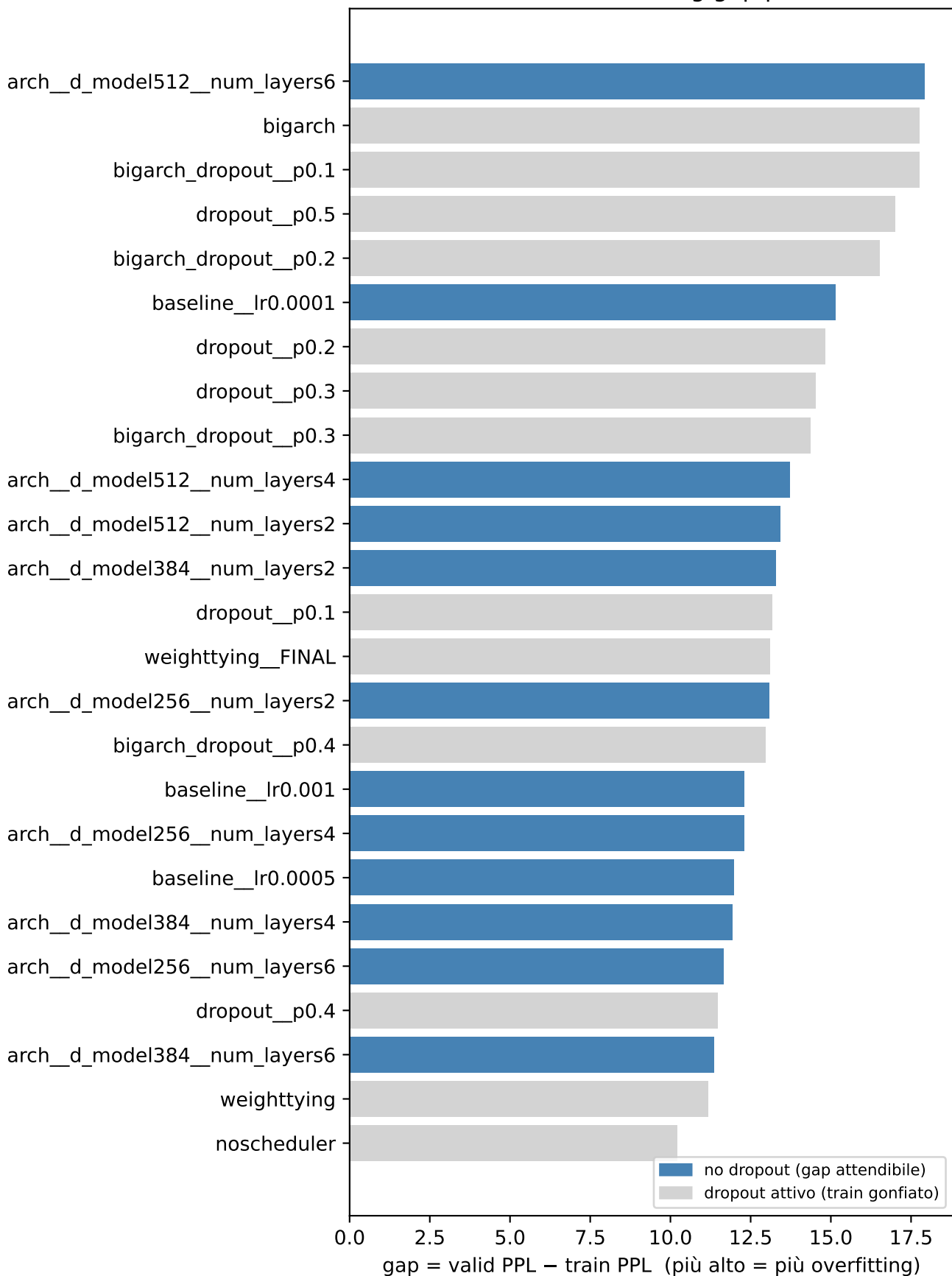
Part 1.A — overfitting gap per run
