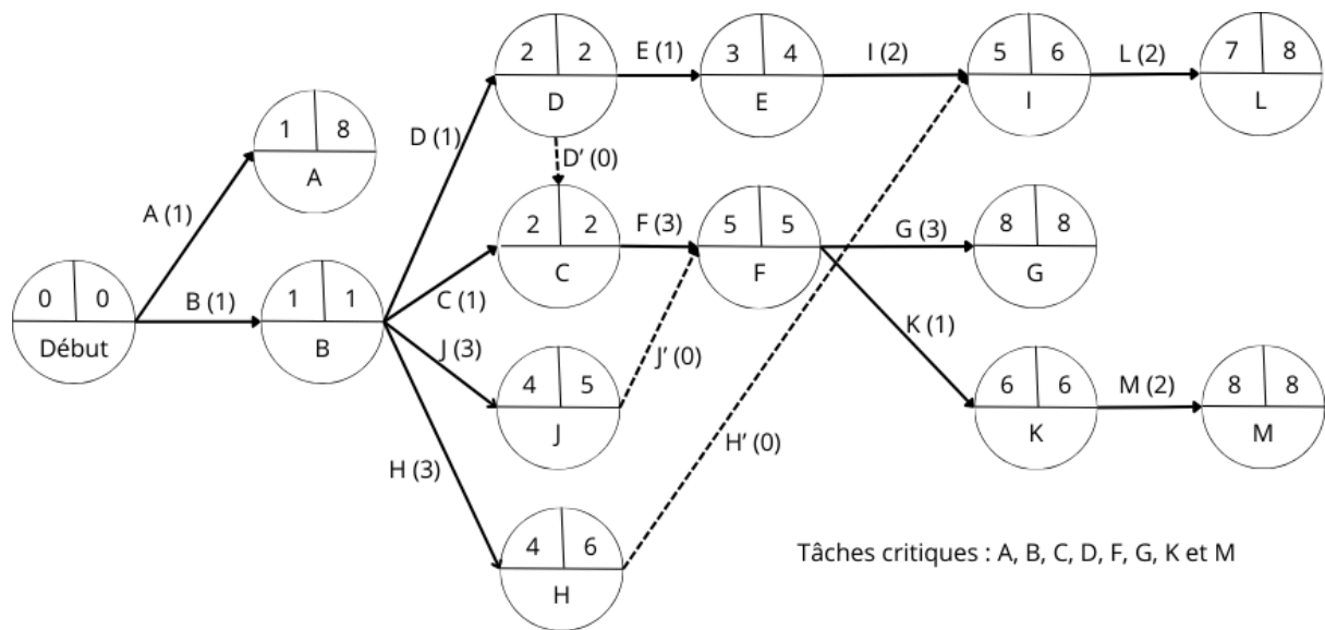
Diagramme de PERT :
