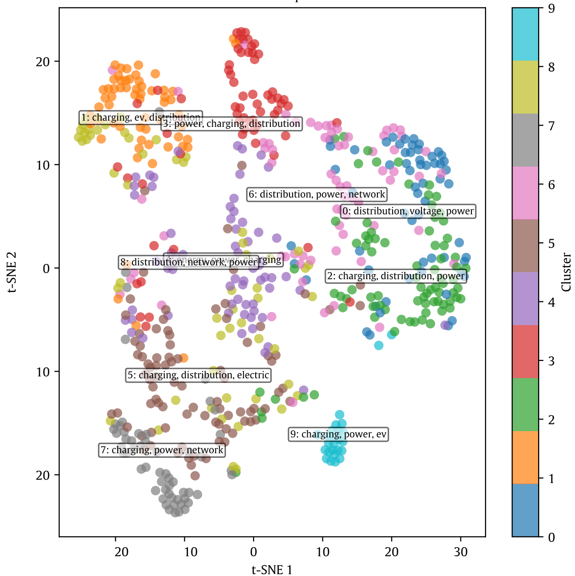
t-SNE Map
