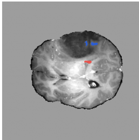
ET error
