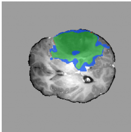
WT error
