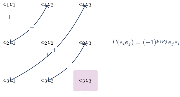
Şekil 6. Süper permütasyon P , V \otimes V bazı üzerinde bir takas: köşegen-dışı çiftler işaretlessiz (+) yer değiştirir, köşegen sabit kalır; tek istisna odd-odd köşesi e_3 e_3 ’tür ( -1 , vurgulu). Klasik takastan tek fark budur.
