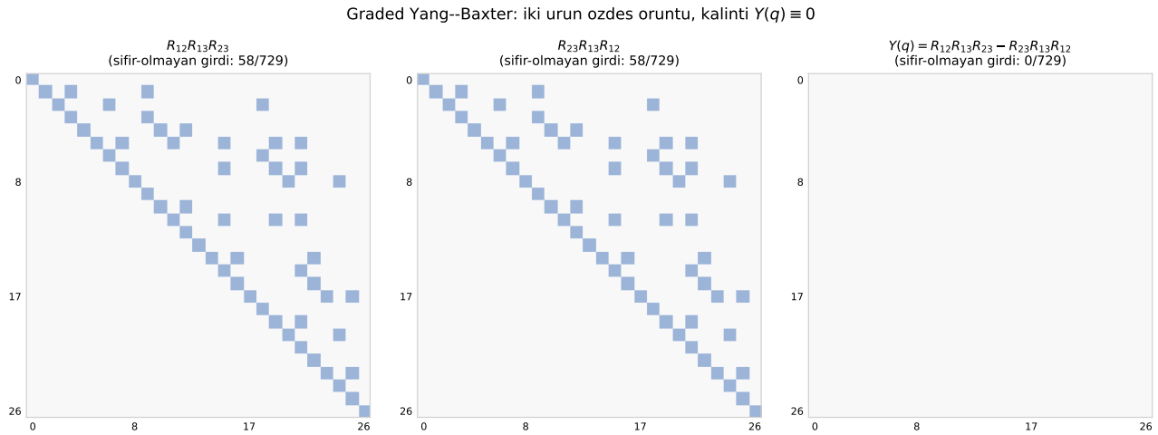
Şekil 8. Graded Yang–Baxter denkleminin iki tarafının 27 \times 27 sıfır-olmayan örüntüleri özdeşdir; kalıntı Y(q) = R_{12}R_{13}R_{23} - R_{23}R_{13}R_{12} tüm 729 girdide sıfırdır ( graded_yang_baxter_residual_GLq21 ).
