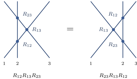
Şekil 3. Kuantum Yang–Baxter denkleminin doğru-diyagramı. Üç doğru ikiyeşerli kesişir; her kesişim bir R_{ij} operatörüdür. İkinci doğruyu R_{13} kesişiminin soluna ya da sağına kaydırmak operatörü değiştirmez: R_{12}R_{13}R_{23} = R_{23}R_{13}R_{12} .
