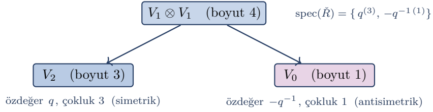
Şekil 4. Örgülü \tilde{R} 'nin spektral ayrışması, V_1 \otimes V_1 = V_2 \oplus V_0 Clebsch–Gordan ayrışımıyla aynıdır. Özdeğer çoklukları doğrudan alt-temsil boyutlarını verir ( R_check_eigenvalues ).
