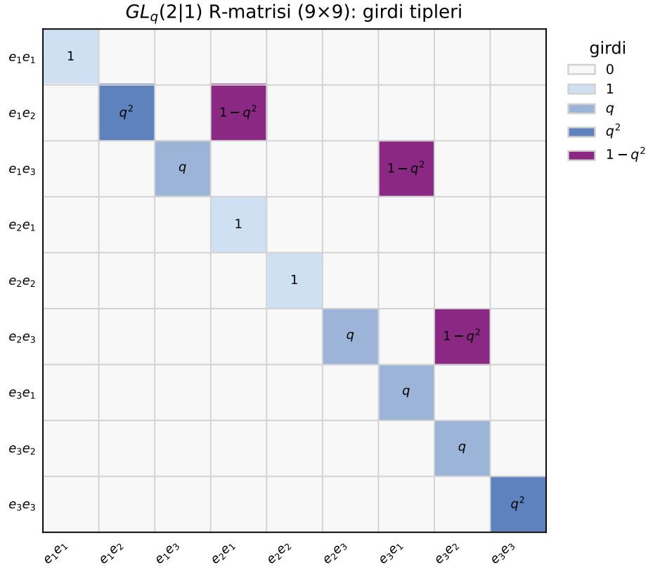
Şekil 5. (9.1) R-matrisinin girdi-tipi haritası ( R_matrix_GLq21 çıktısı). Köşegen q/q^2 terimleri ile köşegen-dışı 1-q^2 “karışım” terimleri açıkça ayrışır; bu seyreklik, 27 \times 27 ve 81 \times 81 yerleşimlerin neden hâlâ hesaplanabilir kaldığını da açıklar.
