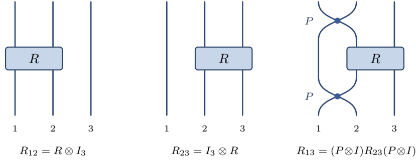
Şekil 7. Üç faktörlü uzayda R_{ij} yerleşimleri. Komşu yerleşimler (R_{12}, R_{23}) basit Kronecker gömmeleridir; uzak yerleşim R_{13} ise süper permütasyon P ile konjugasyon gerektirir — elle takibi en zor olan, bu çalışmada otomatikleştirilen adım.
