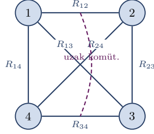
Şekil 9. V^{\otimes 4} yerleşimlerinin K_4 grafiği: altı kenar altı R_{ij} , dört üçgen ( \{1, 2, 3\}, \{1, 2, 4\}, \{1, 3, 4\}, \{2, 3, 4\} ) dört lokal Yang–Baxter kontrolü, ayırık kenar çifti (12) - (34) ise uzak komütativitedir.
