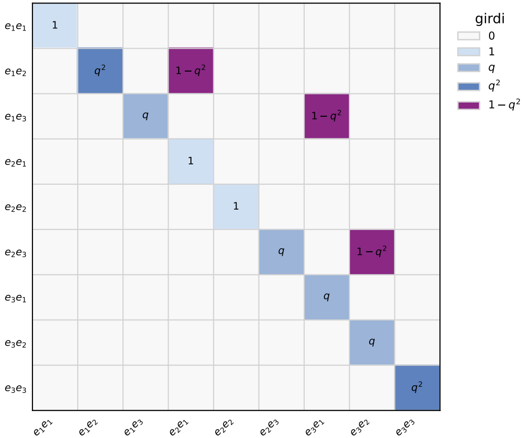
GL_q(2|1) R-matrisi (9×9): girdi tipleri
