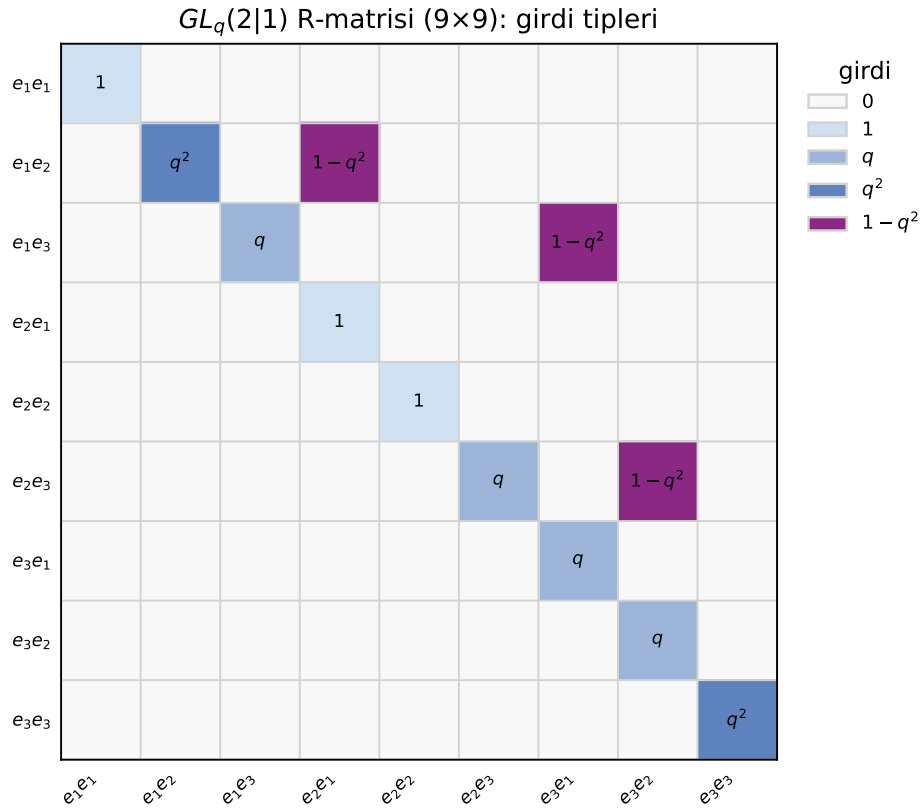
Şekil 5. (9.1) R -matrisinin girdi-tipi haritası ( R_matrix_GLq21 çıktısı). Köşegen q/q^2 terimleri ile köşegen-dışı 1-q^2 “karışım” terimleri açıkça ayrışır; bu seyreklik, 27 \times 27 ve 81 \times 81 yerleşimlerin neden hâlâ hesaplanabilir kaldığını da açıklar.
