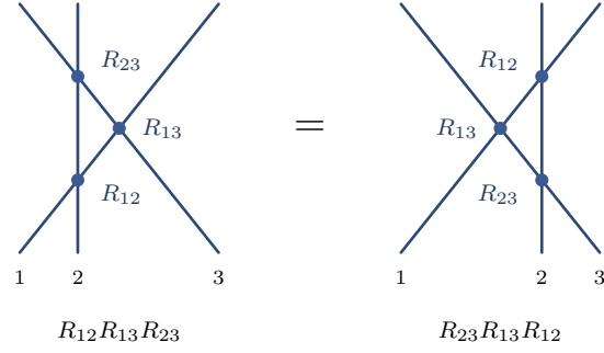
Şekil 3. Kuantum Yang–Baxter denkleminin doğru-diyagramı. Üç doğru ikişerli kesişir; her kesişim bir R_{ij} operatörüdür. İkinci doğruyu R_{13} kesişiminin soluna ya da sağına kaydırmak operatörü değıştirmmez: R_{12}R_{13}R_{23} = R_{23}R_{13}R_{12} .
