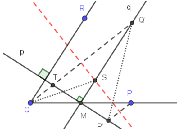
Slika 57: Martinov postopek za trisekcijo kota iz [29, str. 154].
