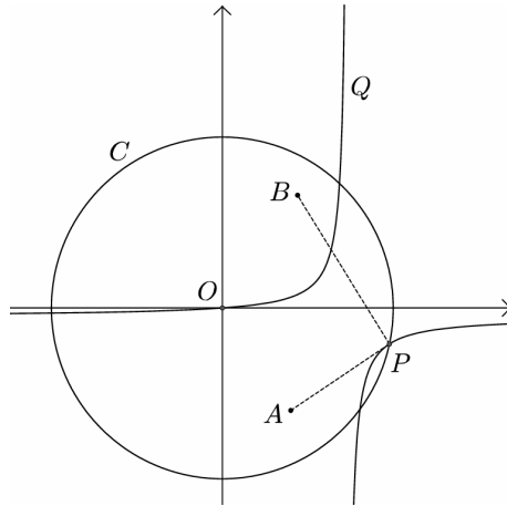
Slika 93: Rešitev Alhazenovega problema kot presečišče krožnice in hiperbole. Vzeto iz [36, str. 39].
