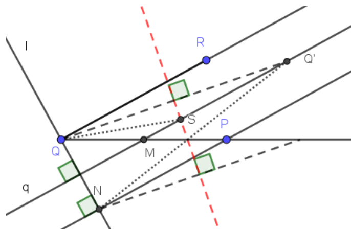
Slika 58: Martinov postopek za trisekcijo kota iz [33, str. 158–159].
