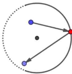
Slika 85: Ptolemajev optični problem.
