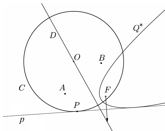
Slika 94: Konstrukcija dotikališča skupne tangente s krožnico. Vzeto iz [36, str. 40].
