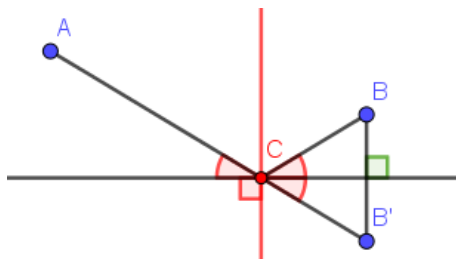
Slika 86: Heronova konstrukcija najkrajše poti od točke A do točke B.
