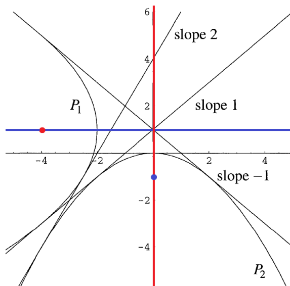
Slika 84: Konstrukcija skupnih tangent na paraboli. Preurejeno iz [7, str. 22].
