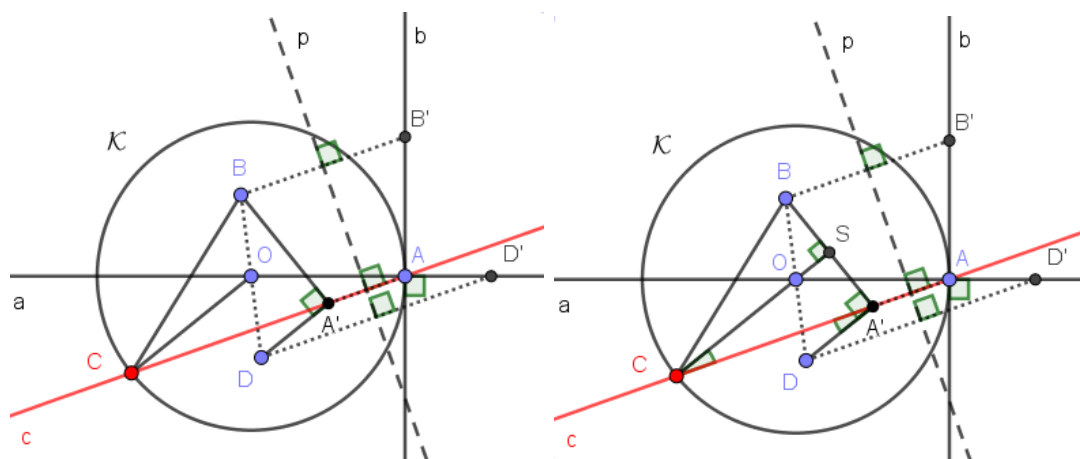
Slika 90: Geometrijski dokaz Scimemijeve konstrukcije
