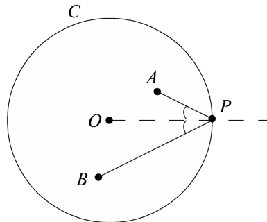
Slika 90: Vprašanje Alhazenovega problema. Vzeto iz [36, str. 37].
