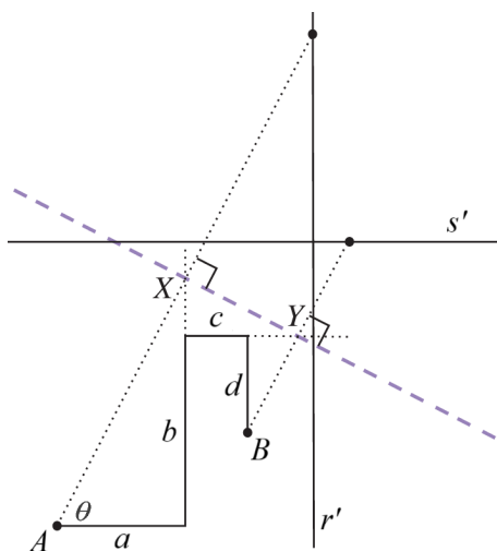
Slika 76: Reševanje enačbe ax^3 + bx^2 + cx + d = 0 . Preurejeno iz [21, str. 42].
