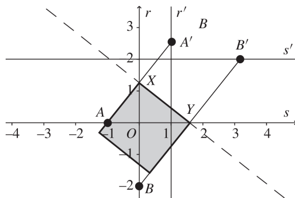
Slika 75: Konstrukcija razdalje |OX| = \sqrt[3]{2} . Vzeto iz [23, str. 310].
