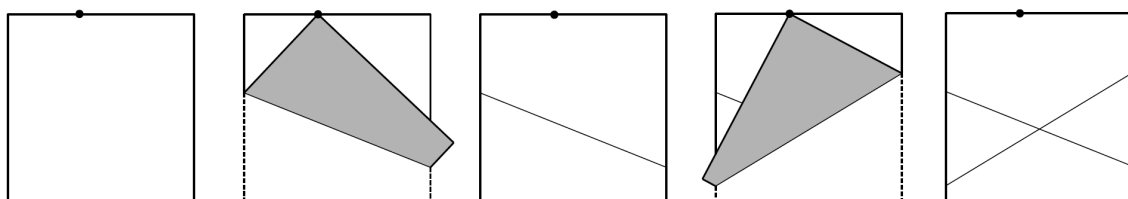
Slika 43: Potek konstrukcije X -pregibov. Predelano iz [14, str. 34].
