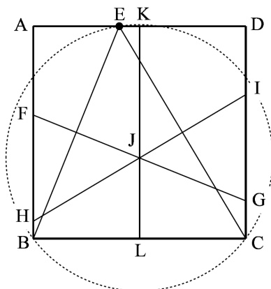
Slika 44: Dokaz, da se X -pregiba in navpična simetrala kvadrata sekajo v isti točki. Vzeto iz [14, str. 38].
