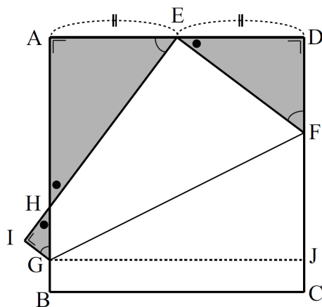
Slika 31: Konstrukcija pregiba iz prvega Hagovega izreka. Vzeto iz [14, str. 4].
