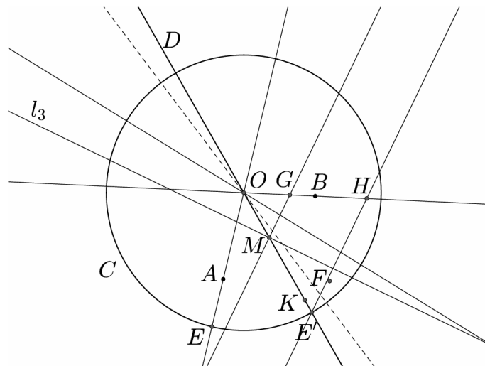
Slika 97: Nishimurijeva origami konstrukcija gorišča F (korak 13). Vzeto iz [36, str. 42].
