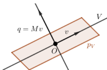
Slika 84: Točka V \in \mathcal{S} rodi tangento p_V z dualom q = Mv .
