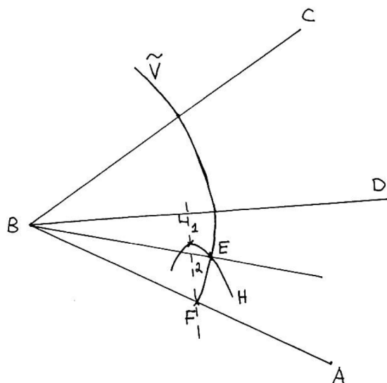
Slika 52: Pappusova trisekcija kota preko stožnic. Vzeto iz [42, str. 7].
