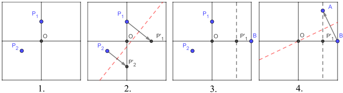
Slika 20: Konstrukcija oglišča A pravielnega sedemkotnika (koraki 1–4).
