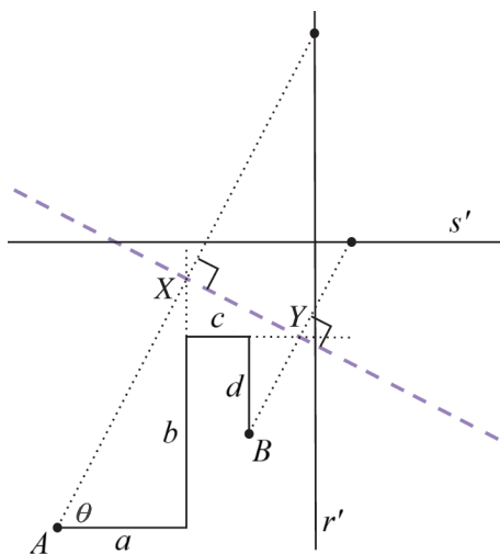
Slika 76: Reševanje enačbe ax^3 + bx^2 + cx + d = 0 . Preurejeno iz [18, str. 42].
