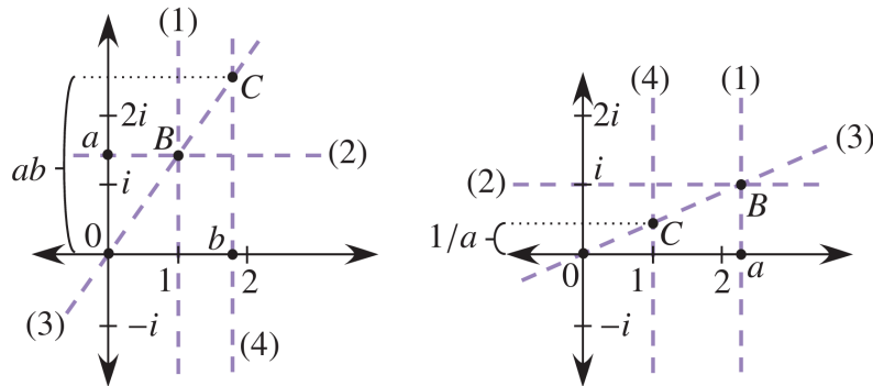
Slika 14: Konstrukcija števil ab in 1/a za neničelna a, b \in \mathbb{C} \cap \mathbb{R} .
