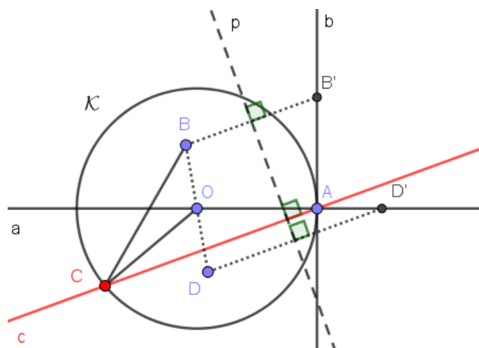
Slika 87: Scimemijeva rešitev Alhazenovega problema, ko točka A leži na krožnici.
