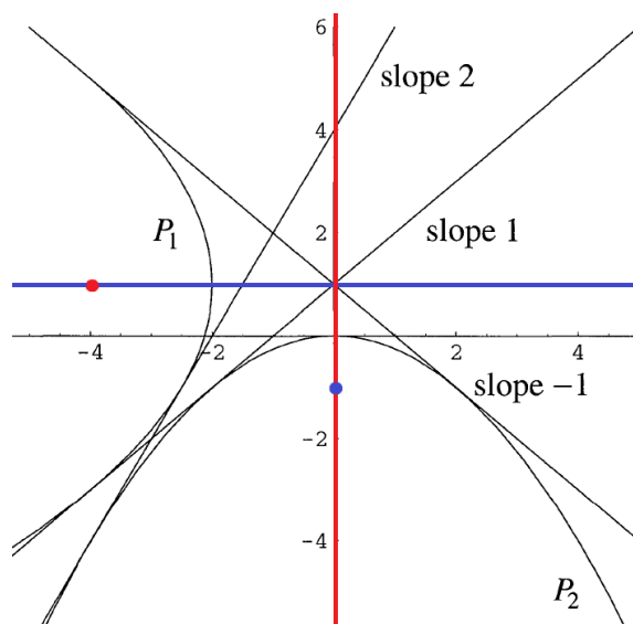
Slika 82: Konstrukcija skupnih tangent na parabolih. Preurejeno iz [7, str. 22].
