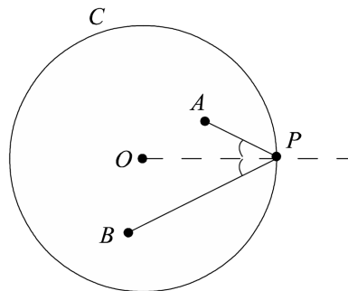
Slika 90: Vprašanje Alhazenovega problema. Vzeto iz [36, str. 37].
