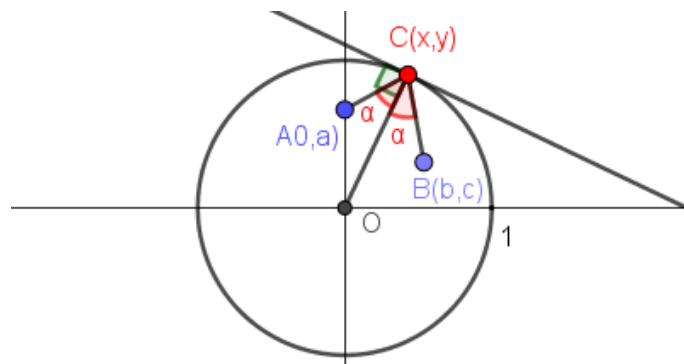
Slika 86: Podlaga za izpeljavo kvartične enačbe za Alhazenov problem.
