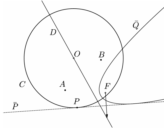
Slika 92: Konstrukcija dotikališča skupne tangente s krožnico. Vzeto iz [36, str. 40].
