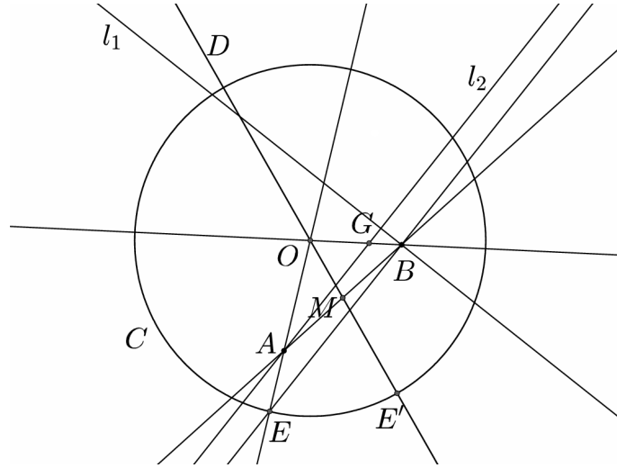
Slika 93: Nishimurijeva origami konstrukcija do koraka 8. Vzeto iz [36, str. 41].
