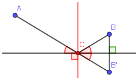
Slika 84: Heronova konstrukcija najkrajše poti od točke A do točke B.
