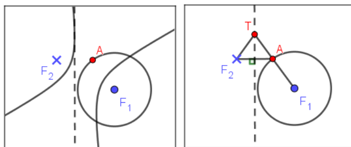
Slika 66: Dokaz tangenčnosti pregibov na hiperbolo.
