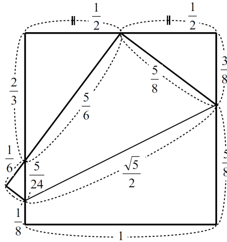
Slika 32: Dolžine daljic po prvem Hagovem izreku. Vzeto iz [14, str. 7].
