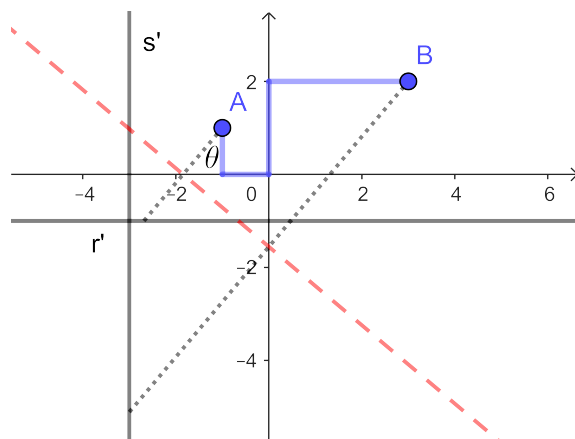
Slika 79: Hatorijeva konstrukcija za enačbo x^3 - x^2 + 2x + 3 = 0 .
