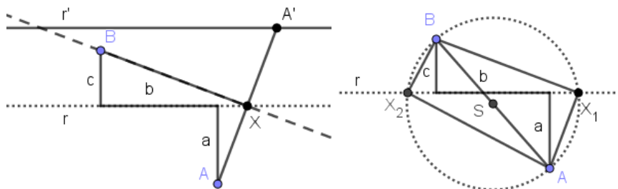
Slika 80: Lillova metoda z operacijo O6 (levo) in Talesovim izrekom (desno).
