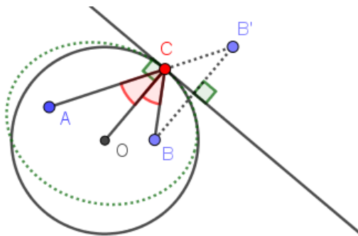
Slika 88: Ena od rešitev Alhazenovega problema v splošnem.
