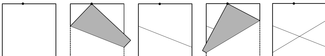
Slika 43: Potek konstrukcije X -pregibov. Predelano iz [13, str. 34].
