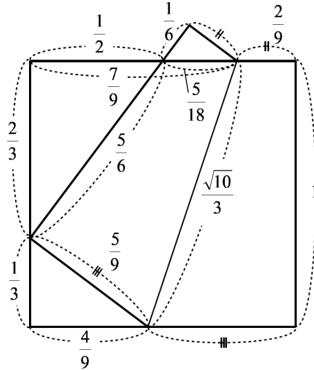
Slika 37: Dolžine daljic po tretjem Hagovem izreku. Vzeto iz [13, str. 19].
