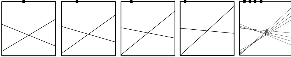
Slika 45: Primeri X -pregibov in njihova unija. Predelano iz [13, str. 36].
