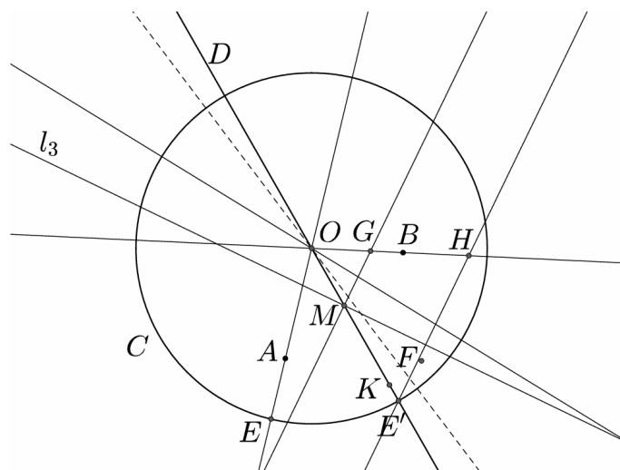
Slika 97: Nishimurijeva konstrukcija gorišča F (korak 13). Vzeto iz [32, str. 42].
