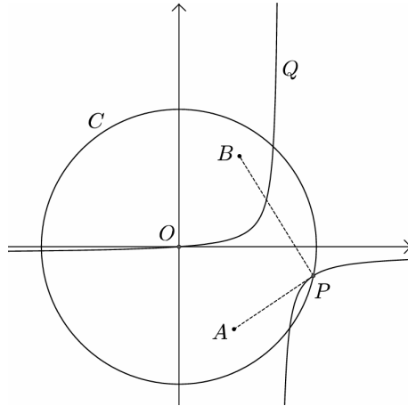
Slika 94: Rešitev Alhazenovega problema kot presečišče krožnice in hiperbole.
