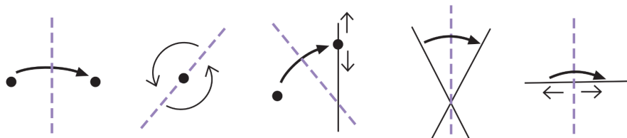
Slika 1: Vsi pregibi točk ali premic na točko ali premico. Vzeto iz [18, str. 25].
