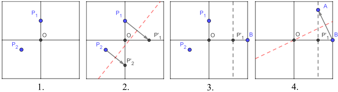
Slika 20: Konstrukcija oglišča A pravilnega sedemkotnika (koraki 1–4).
