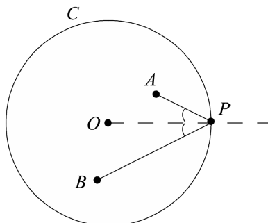
Slika 93: Vprašanje Alhazenovega problema. Vzeto iz [32, str. 37].
