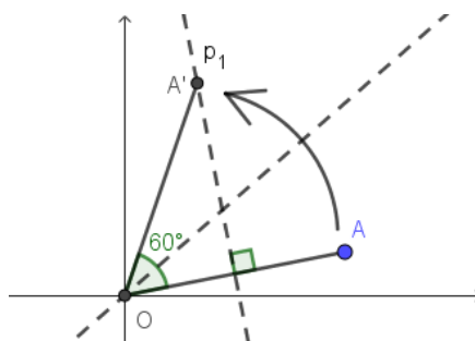
Slika 16: Rotacija točke za kot 60^\circ okoli izhodišča.
