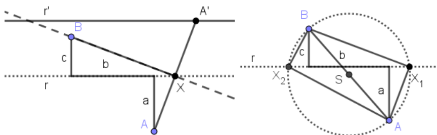
Slika 80: Lillova metoda z operacijo O6 (levo) in Talesovim izrekom (desno).
