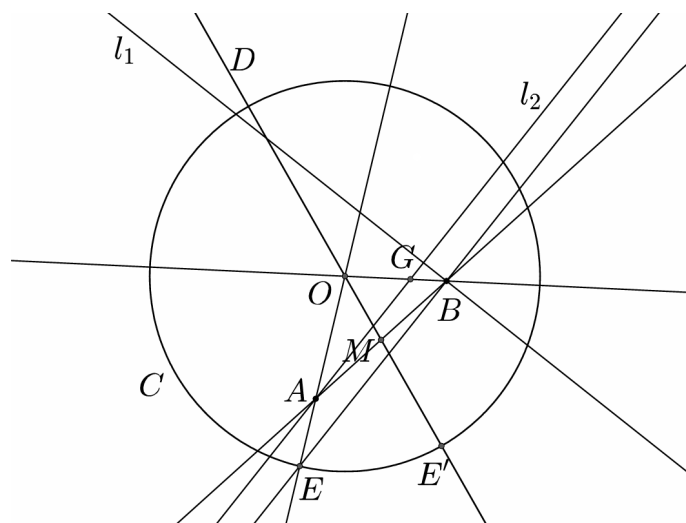
Slika 96: Nishimurijeva origami konstrukcija do koraka 8. Vzeto iz [32, str. 41].
