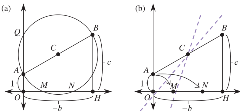
Slika 69: Reševanje enačbe x^2 + bx + c = 0 . Preurejeno iz [18, str. 38].
